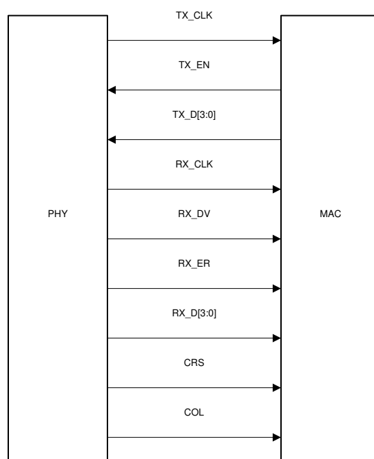
图 8-4. MII Signaling
