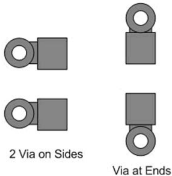
图 9-6. 去耦过孔放置方式
