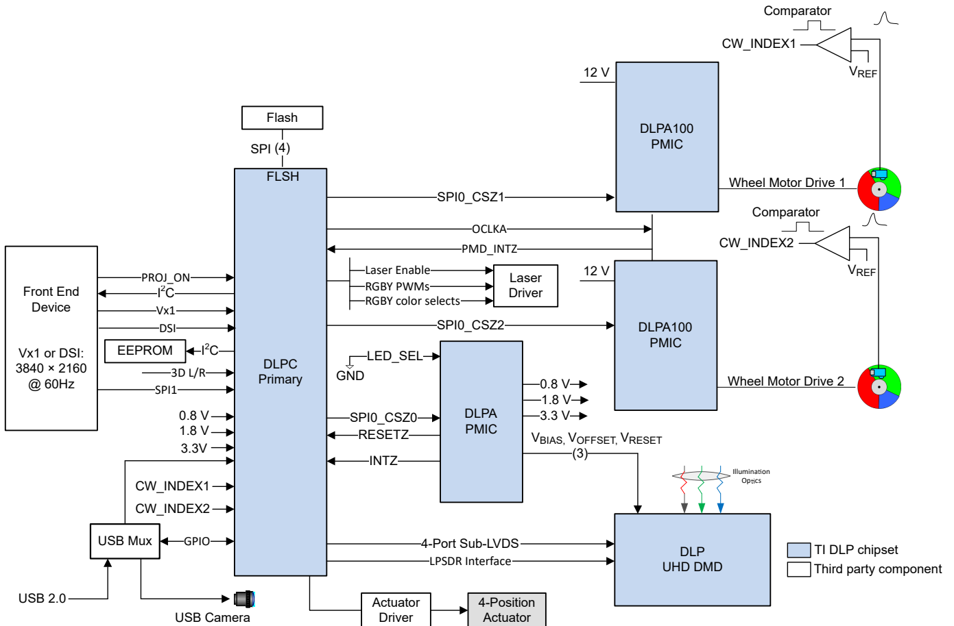
图 6-2. 激光荧光功能方框图
