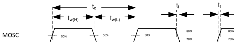
图 5-1. System Oscillators
