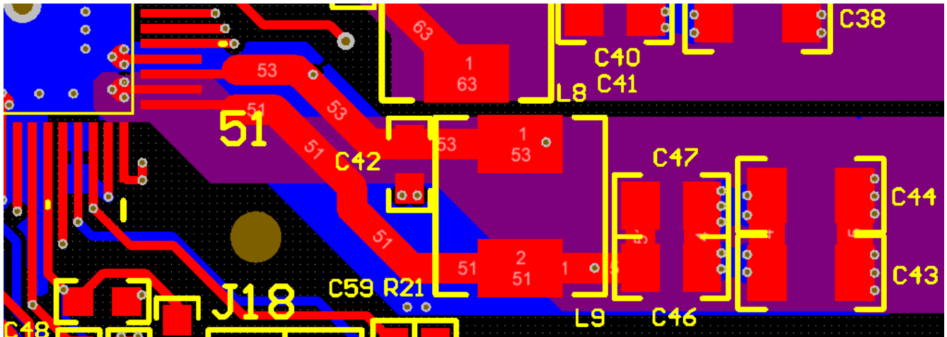
图 7-7. 实用布局
