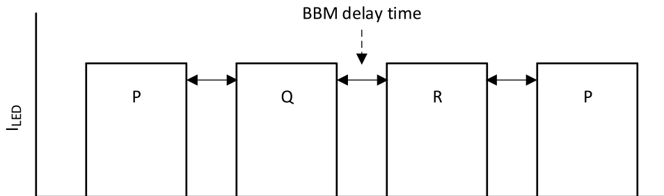
图 8-8. BBM Timing
