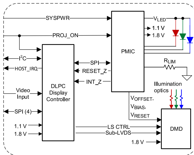
典型简化系统图
