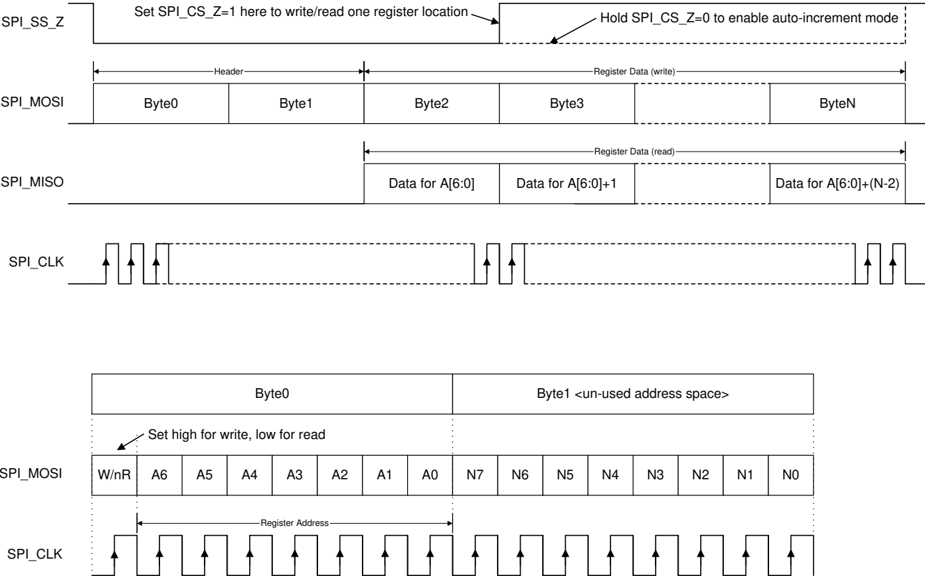
图 8-24. SPI Protocol
