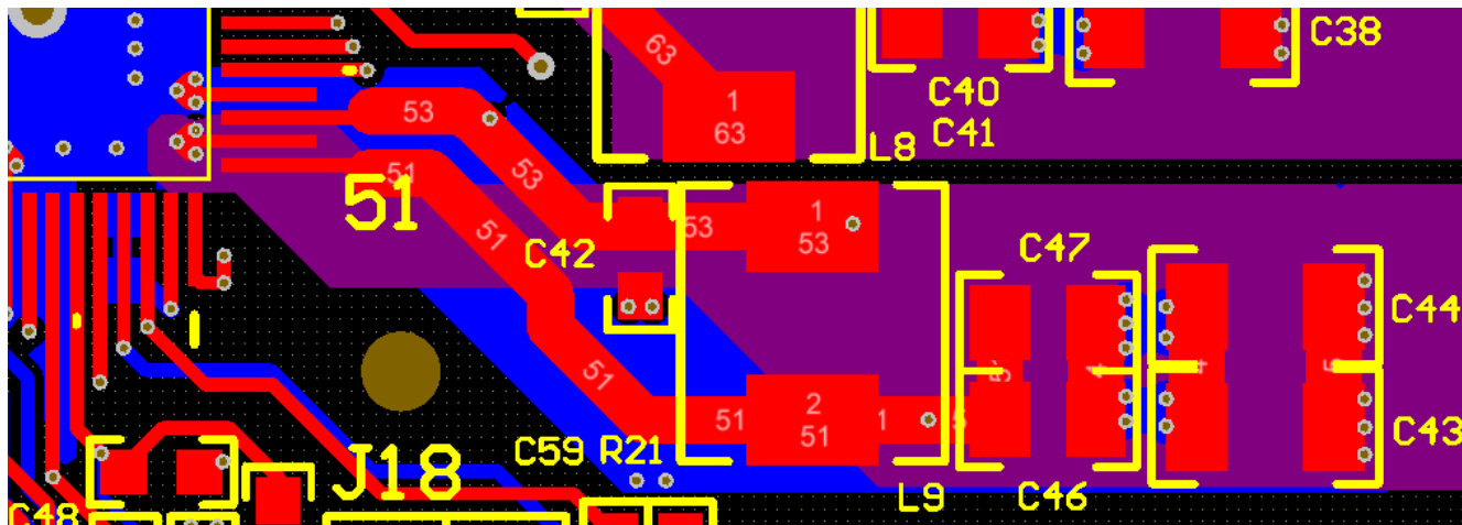
图 11-2. Practical Layout
