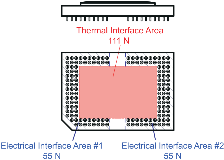
图 6-10. System Interface Loads
