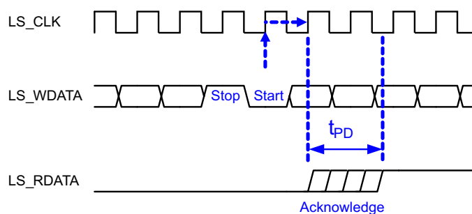
图 5-13. LPSDR 读取
