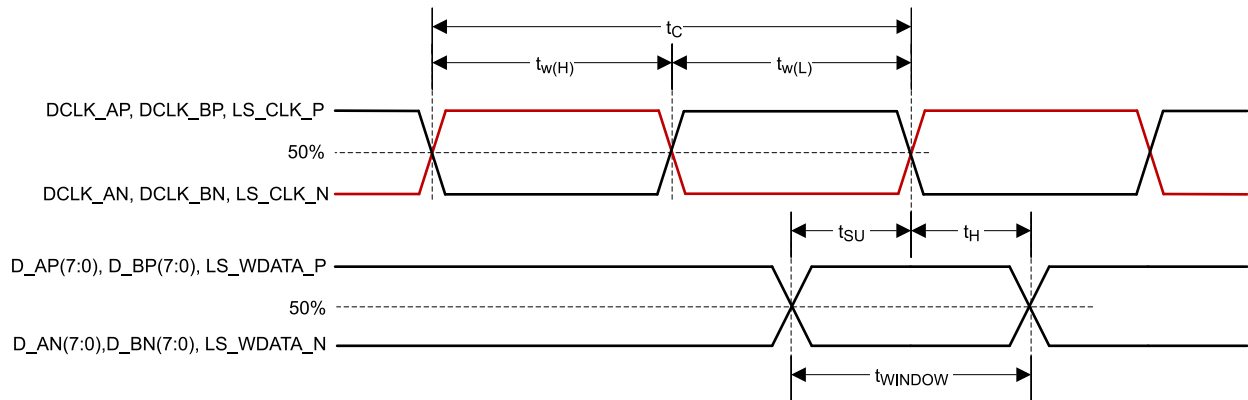
图 5-4. SubLVDS Switching Parameters
