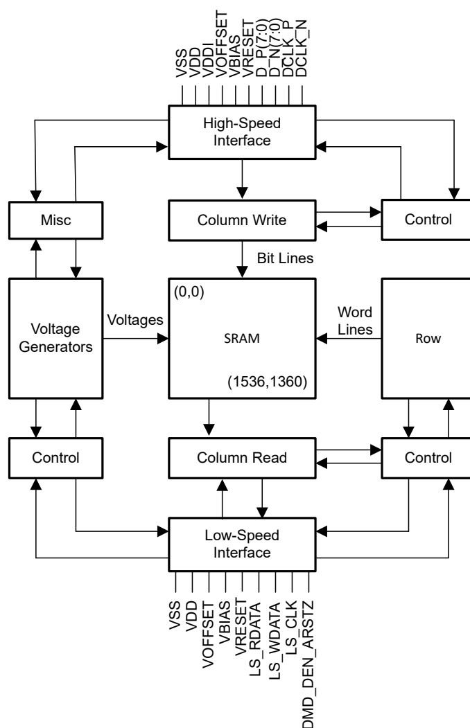
图 6-1. 功能方框图
