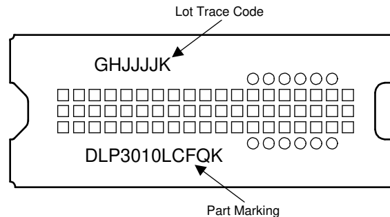
图 11-2. DMD Marking
