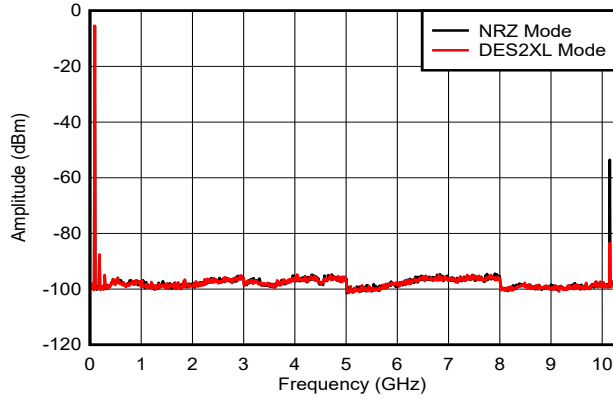
图 6-8. f_{\text{OUT}} = 97\text{MHz} ，0dBFS
