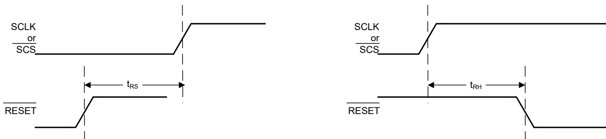
图 6-5. RESET 时序图
