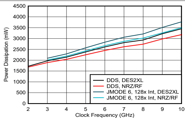
图 6-45. 功率损耗与时钟频率和数字模式间的关系
