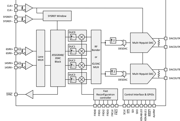
方框图（双通道器件）
