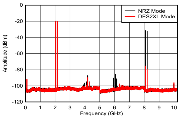
图 6-33. 双音， f_{\text{OUT}} = 2097\text{MHz} ，-6dBFS
