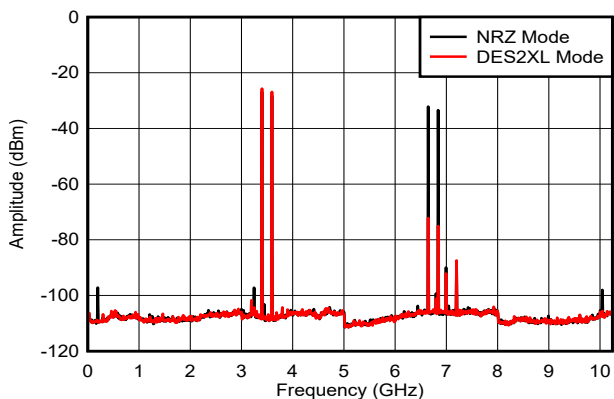
图 6-35. 双音， f_{\text{OUT}} = 3497\text{MHz} ，0dBFS
