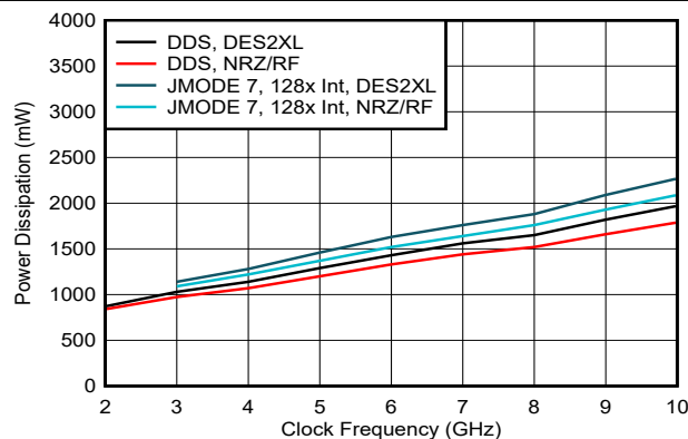
图 6-44. 功率损耗与时钟频率和数字模式间的关系
