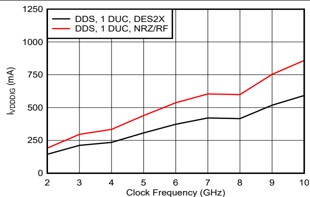
图 6-56. VDDDIG 电流与时钟频率和数字模式间的关系
