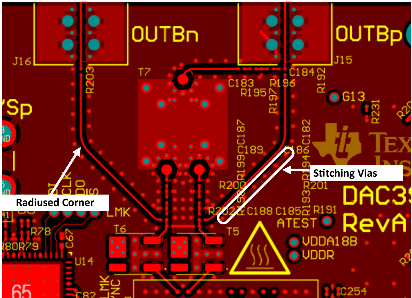
图 8-23. 高速信号布线旁边的半径角和拼接过孔
