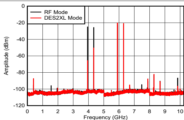
图 6-39. 双音， f_{\text{OUT}} = 6097\text{MHz} ，-6dBFS
