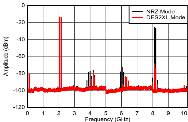
图 6-32. 双音， f_{\text{OUT}} = 2097\text{MHz} ，0dBFS
