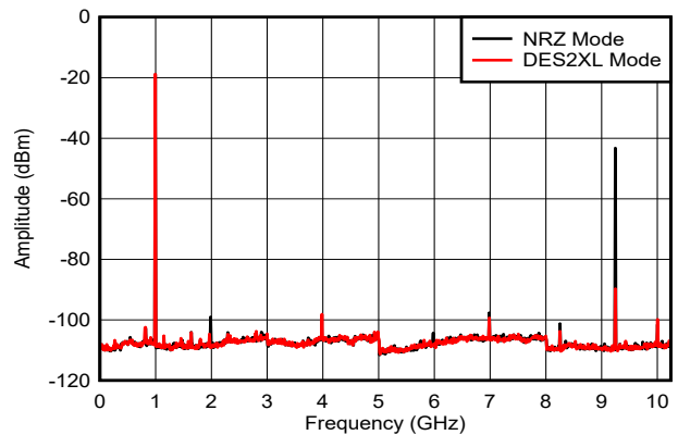
图 6-11. f_{\text{OUT}} = 997\text{MHz} ，0dBFS
