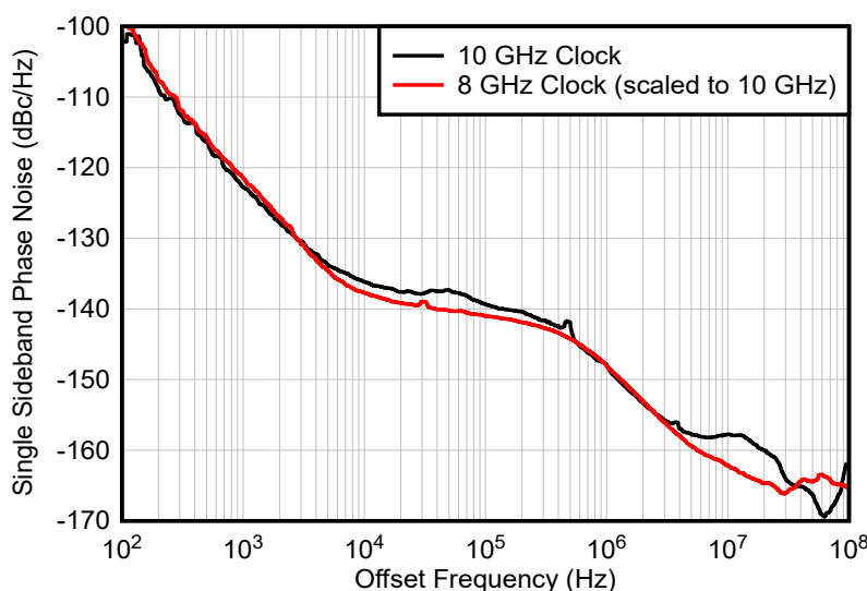
图 8-12. 8GHz 和 10GHz 时钟相位噪声
