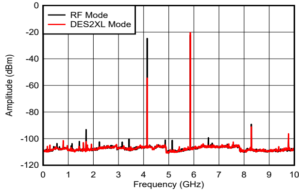
图 6-20. f_{\text{OUT}} = 5997\text{MHz} ，0dBFS
