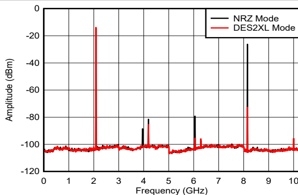
图 6-15. f_{\text{OUT}} = 2097\text{MHz} ，-6dBFS
