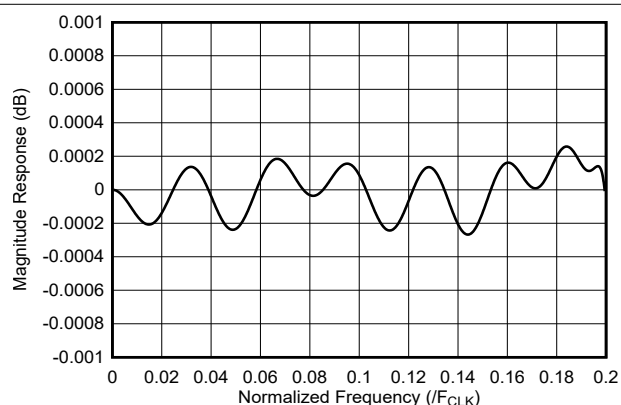
图 7-15. 2 倍内插滤波器通带响应
