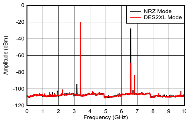
图 6-17. f_{\text{OUT}} = 3497\text{MHz} ，0dBFS
