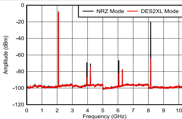
图 6-14. f_{\text{OUT}} = 2097\text{MHz} ，0dBFS
