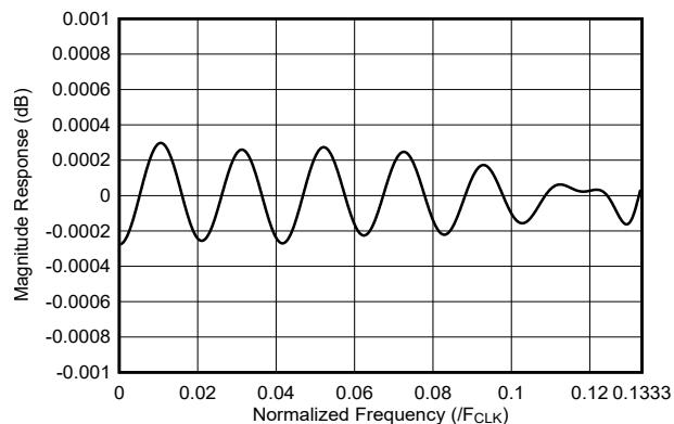
图 7-17. 3 倍内插滤波器通带响应
