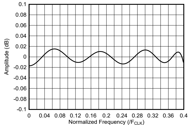
图 7-49. DES 内插器频率响应 (通带)
