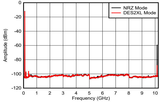
图 6-9. f_{\text{OUT}} = 97\text{MHz} ，-6dBFS
