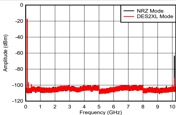
图 6-27. 双音， f_{\text{OUT}} = 97\text{MHz} ，-6dBFS
