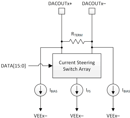
图 7-11. 模拟输出结构
