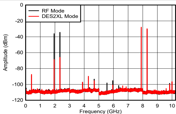
图 6-43. 双音， f_{\text{OUT}} = 8097\text{MHz} ，-12dBFS
