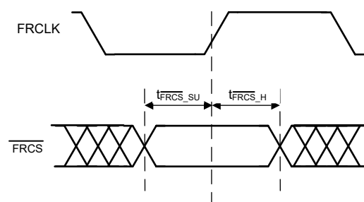
图 6-7. \overline{\text{FRCS}} 时序图
