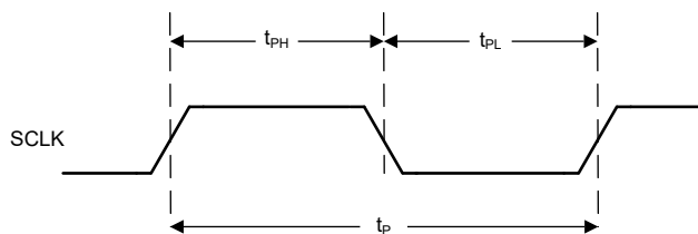
图 6-1. SPI 时钟时序图
