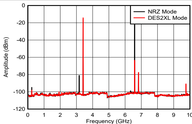
图 6-16. f_{\text{OUT}} = 2097\text{MHz} ，-12dBFS
