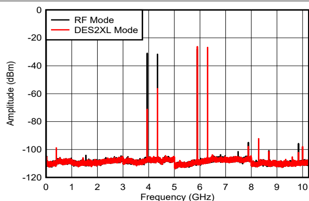
图 6-38. 双音， f_{\text{OUT}} = 6097\text{MHz} ，0dBFS
