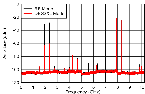
图 6-42. 双音， f_{\text{OUT}} = 8097\text{MHz} ，-6dBFS
