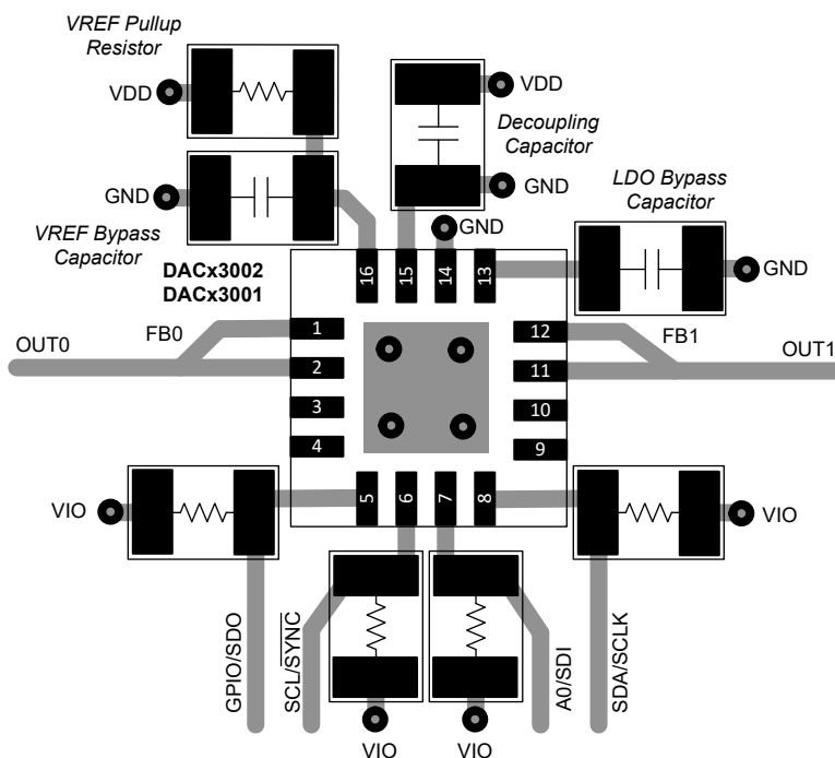
图 10-1. Layout Example
