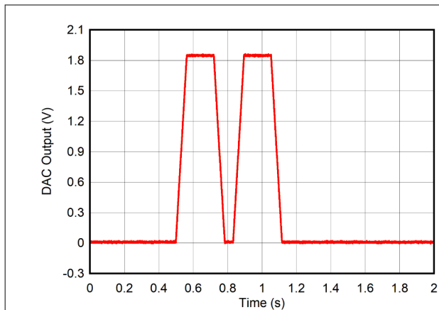
图 9-8. Low Priority Alarm
