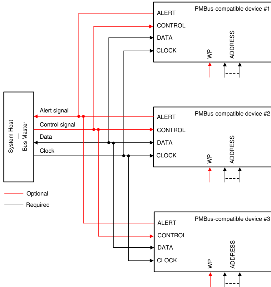
图 8-2. PMBus Connections
