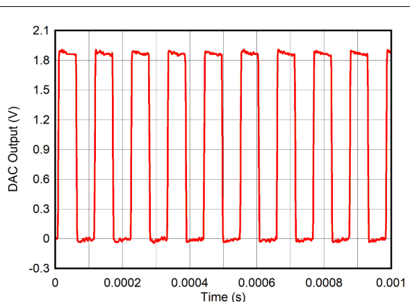
图 9-11. Pulse Frequency
