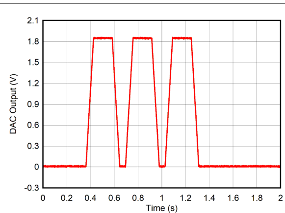
图 9-9. Medium Priority Alarm
