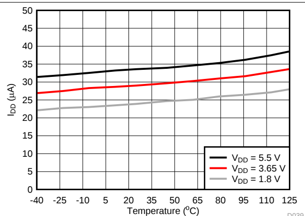
图 26. 电源电流与温度间的关系
