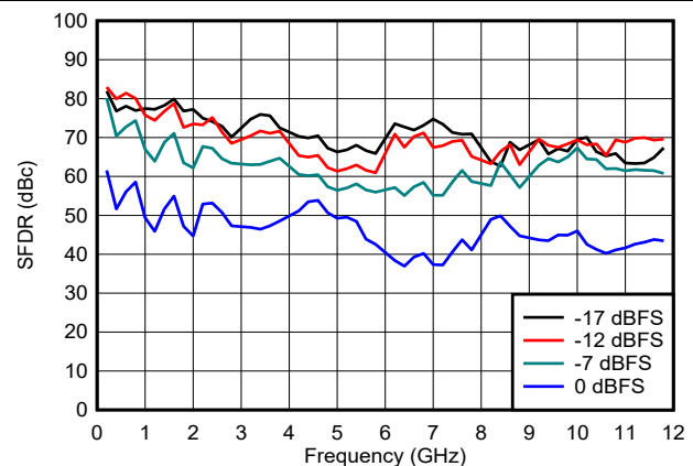
图 6-95. NRZ/RF 模式下 SFDR 与频率和数字振幅间的关系
