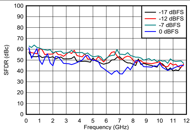
图 6-94. NRZ/RF 模式下 SFDR 与频率和数字振幅间的关系
