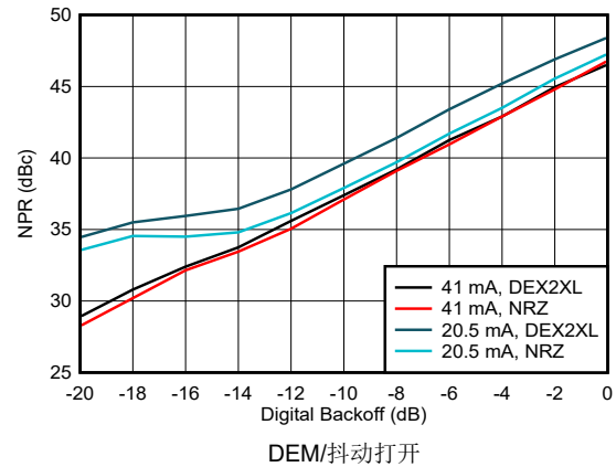
图 6-188. 噪声功率比与数字退避：第一奈奎斯特区域
