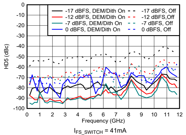
图 6-179. NRZ/RF 模式下 HD5 与频率和数字振幅间的关系
