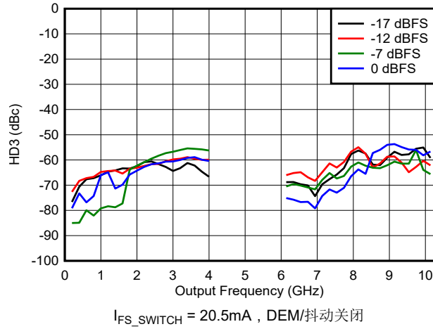
图 6-180. DES2X 模式下 HD3 与频率和数字振幅间的关系
