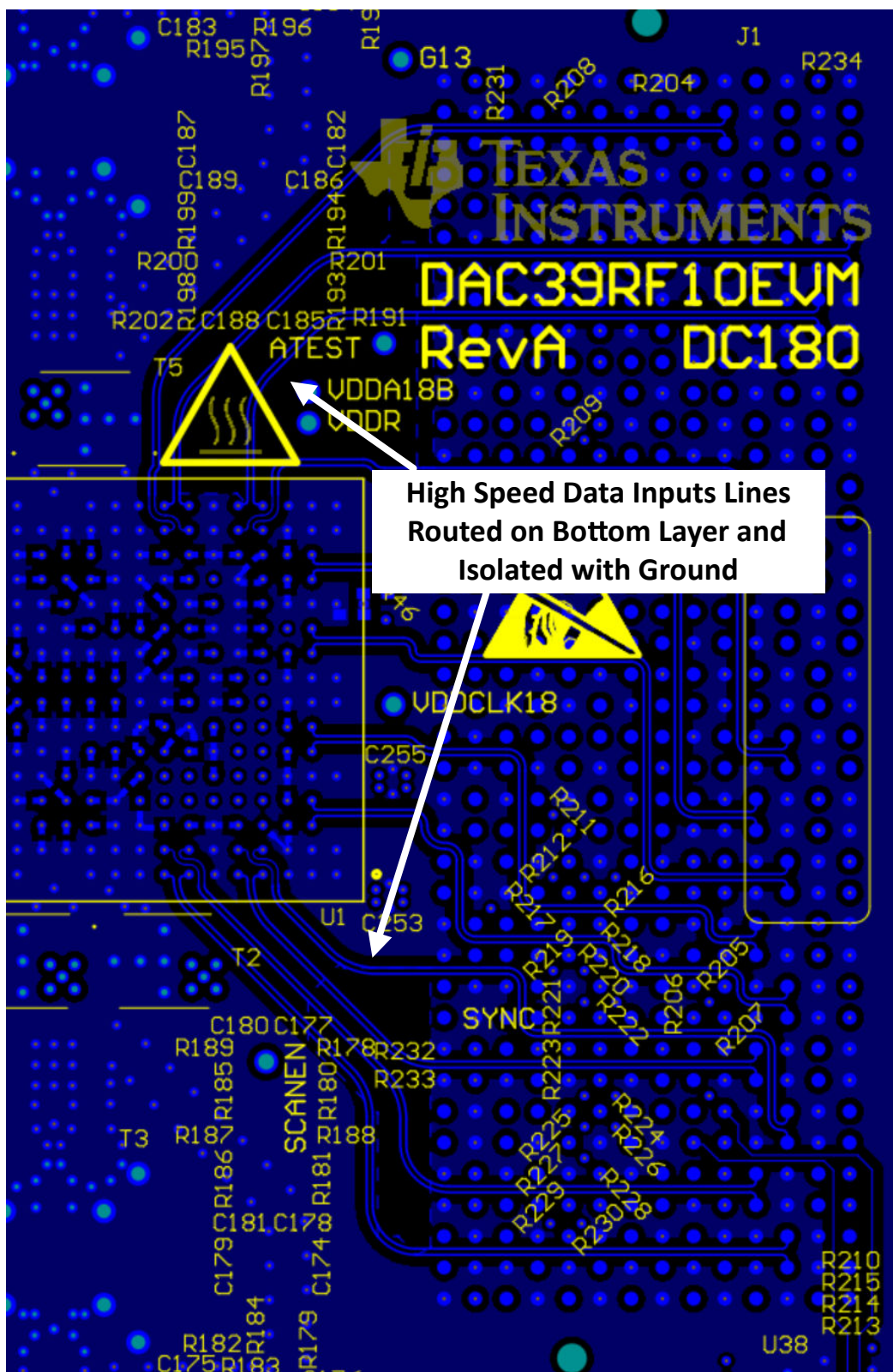
图 9-28. 具有接地隔离的串行器/解串器底层布线
