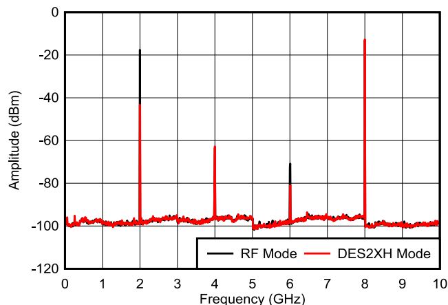
图 9-4. DES2XH 和 RF 模式的输出频谱比较
