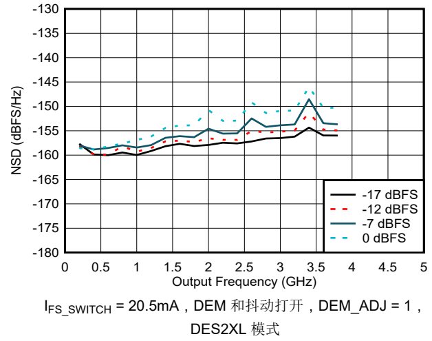
图 6-75. NSD 与输出频率和数字振幅间的关系
