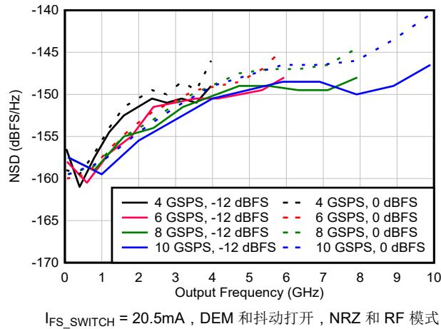
图 6-78. NSD 与输出频率和采样速率间的关系
