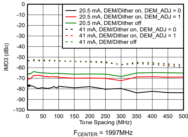
图 6-140. NRZ 模式下 IMD3 与频率间隔间的关系
