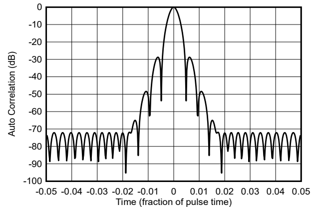
图 9-16. NLFM 线性调频脉冲的自动关联
