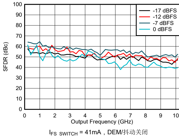
图 6-118. NRZ/RF 模式下 SFDR 与频率和数字振幅间的关系
