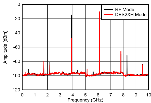
图 6-31. f_{\text{OUT}} = 6097\text{MHz} ，0dBFS
