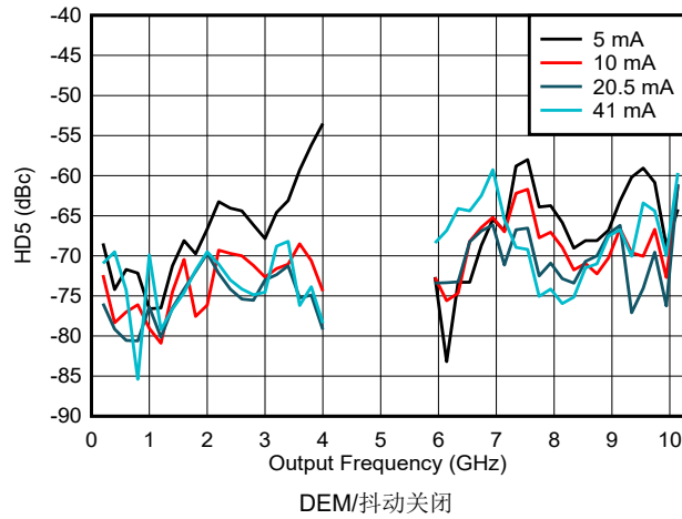
图 6-194. DES2X 模式下 HD5 与频率和输出电流间的关系
