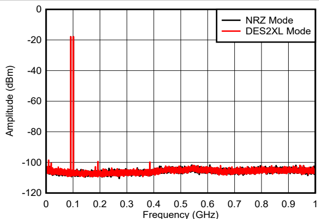
图 6-38. 双音， f_{\text{OUT}} = 97\text{MHz} ，0dBFS (0GHz 至 1GHz)
