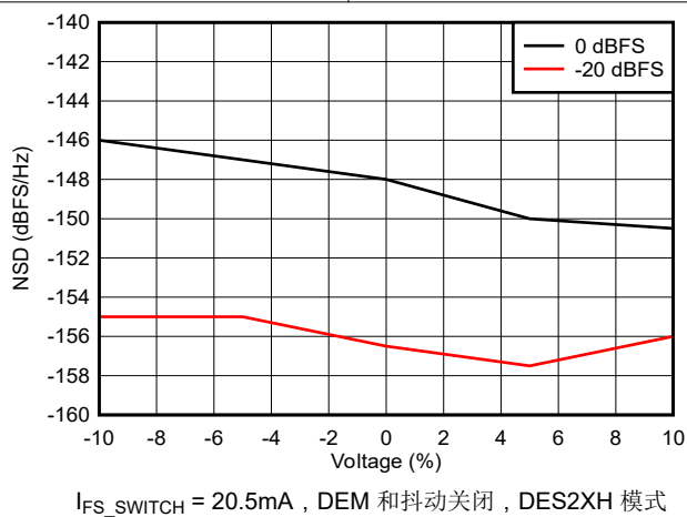
图 6-88. NSD 与电源电压间的关系
