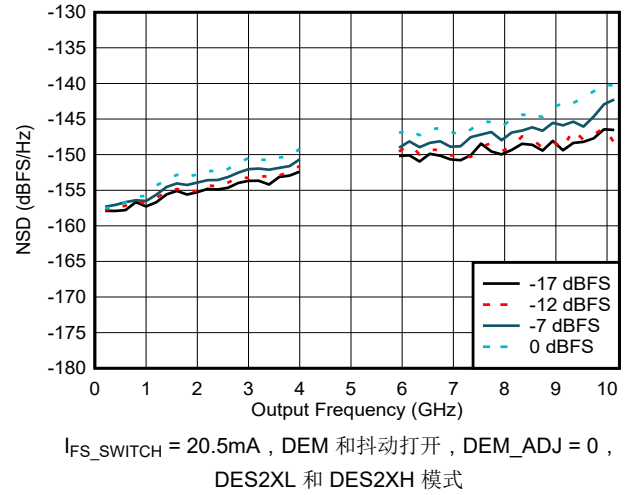
图 6-73. NSD 与输出频率和数字振幅间的关系
