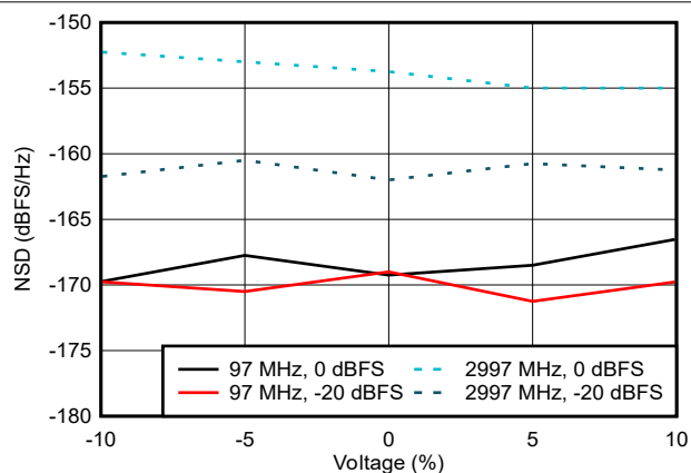
图 6-87. NSD 与电源电压间的关系
