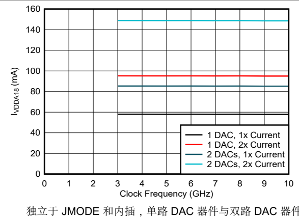
图 6-94. VDDA18 电流与时钟频率和 DAC 模式间的关系
