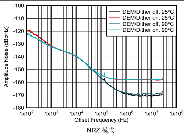
图 6-224. 1GHz 条件下振幅噪声与偏移频率和温度间的关系
