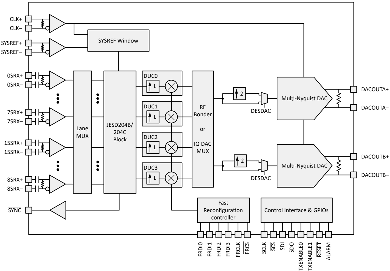
图 7-1. 双通道器件
