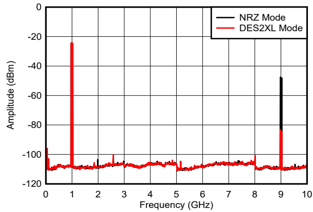
图 6-45. 双音， f_{\text{OUT}} = 997\text{MHz} ， -12\text{dBFS}
