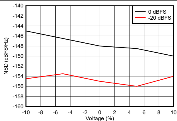
图 6-86. NSD 与电源电压间的关系
