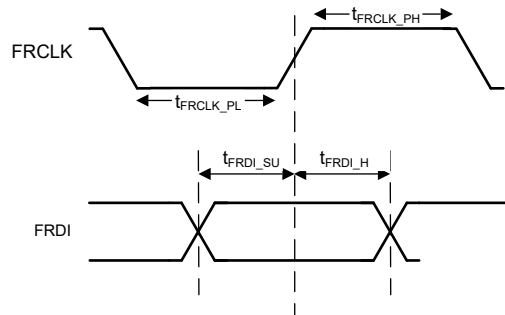
图 6-6. FRDI 时序图
