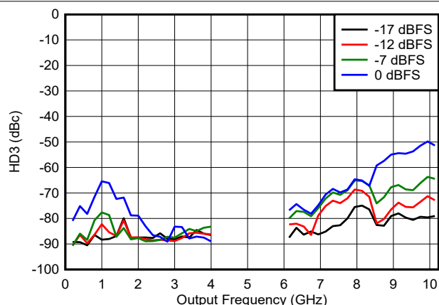
图 6-181. DES2X 模式下 HD3 与频率和数字振幅间的关系
