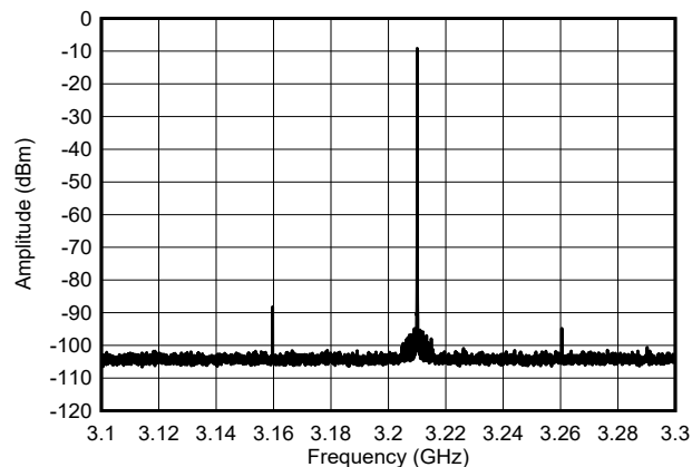
图 9-19. f_{OUT} = 3.211\text{GHz} 时的带内单音频谱
