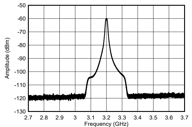
图 9-18. 1GHz 频率下的 NLFM 线性调频脉冲输出频谱
