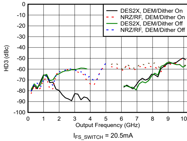
图 6-110. HD3 与频率和模式间的关系
