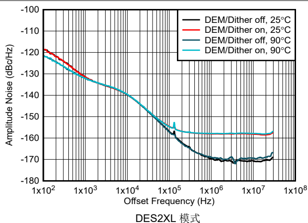
图 6-225. 1GHz 条件下振幅噪声与偏移频率和温度间的关系
