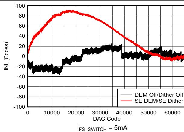
图 6-14. INL 与 DAC 代码间的关系：5mA
