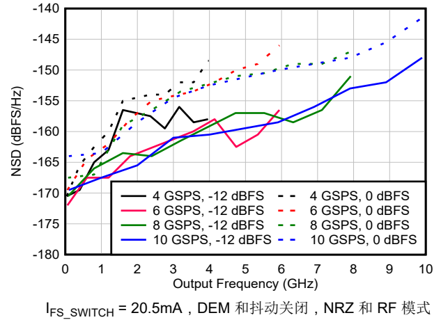
图 6-77. NSD 与输出频率和采样速率间的关系
