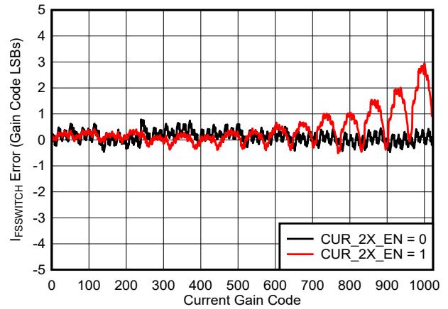
图 6-17. I_{\text{FS\_SWITCH}} 误差与增益代码间的关系
