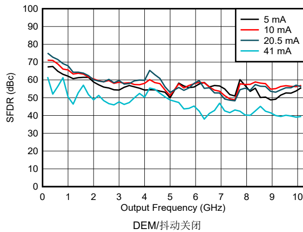
图 6-112. NRZ/RF 模式下 SFDR 与频率和输出电流间的关系
