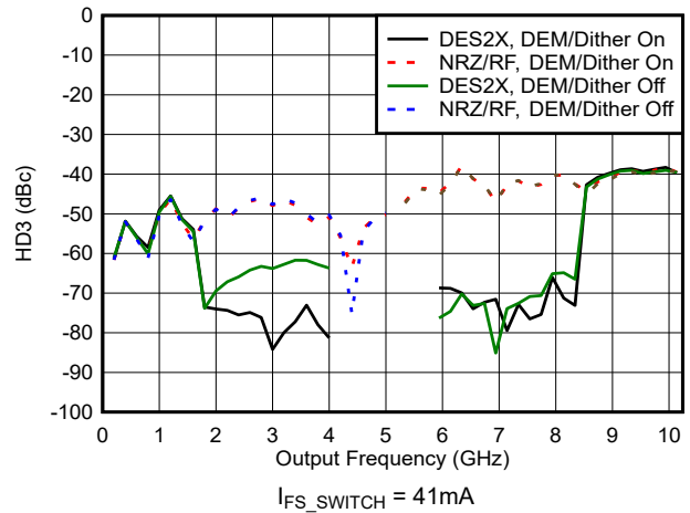
图 6-111. HD3 与频率和模式间的关系
