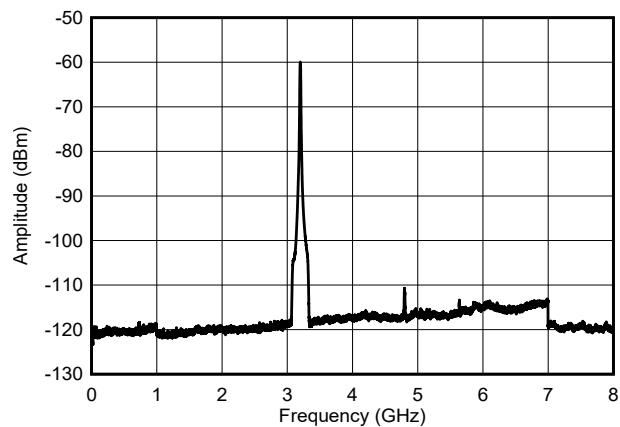
图 9-17. 0GHz 至 8GHz 频率下的 NLFM 线性调频脉冲输出频谱
