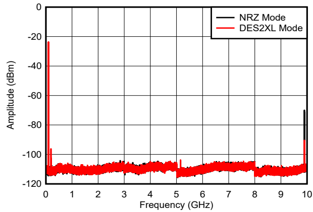
图 6-41. 双音， f_{\text{OUT}} = 97\text{MHz} ， -12\text{dBFS} ( 0 - f_{\text{CLK}} )
