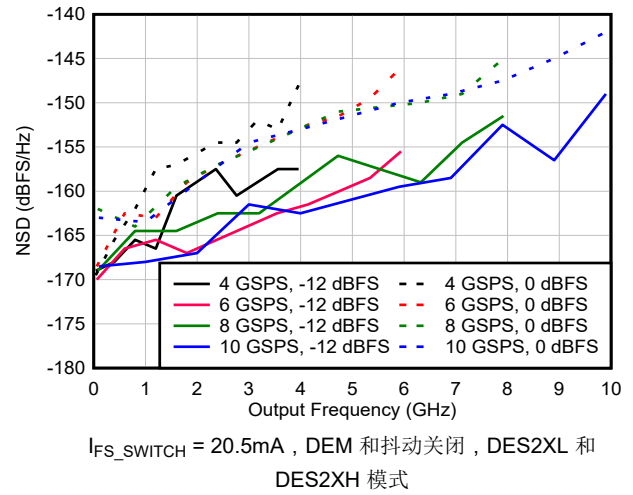
图 6-79. NSD 与输出频率和采样速率间的关系
