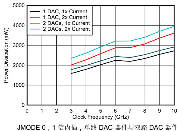
图 6-93. 功率损耗与时钟频率和 DAC 模式间的关系
