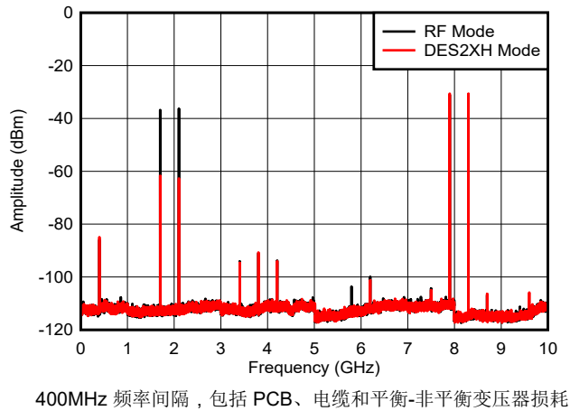
图 6-57. 双音， f_{\text{OUT}} = 7997\text{MHz} ，-12dBFS
