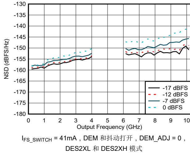
图 6-74. NSD 与输出频率和数字振幅间的关系
