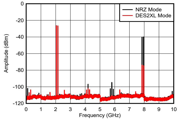
图 6-46. 双音， f_{\text{OUT}} = 2097\text{MHz} ， 0\text{dBFS}
