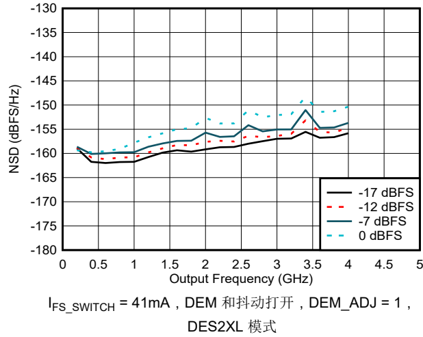
图 6-76. NSD 与输出频率和数字振幅间的关系
