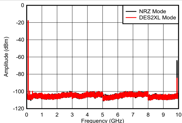
图 6-37. 双音， f_{\text{OUT}} = 97\text{MHz} ，0dBFS (0 - f_{\text{CLK}} )
