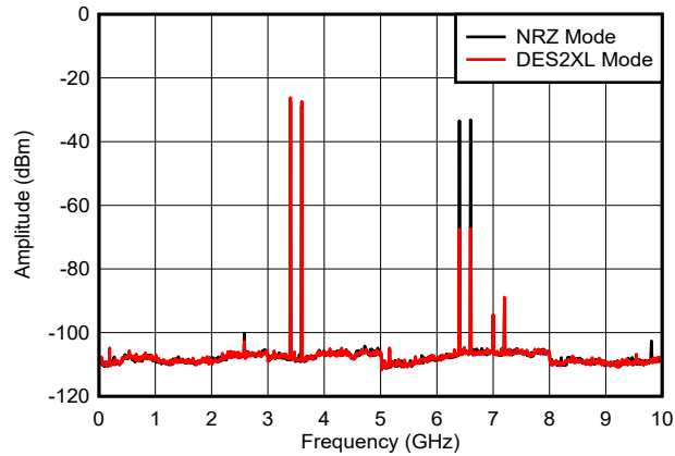
图 6-49. 双音， f_{\text{OUT}} = 3497\text{MHz} ，0dBFS
