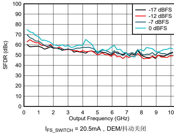
图 6-116. NRZ/RF 模式下 SFDR 与频率和数字振幅间的关系
