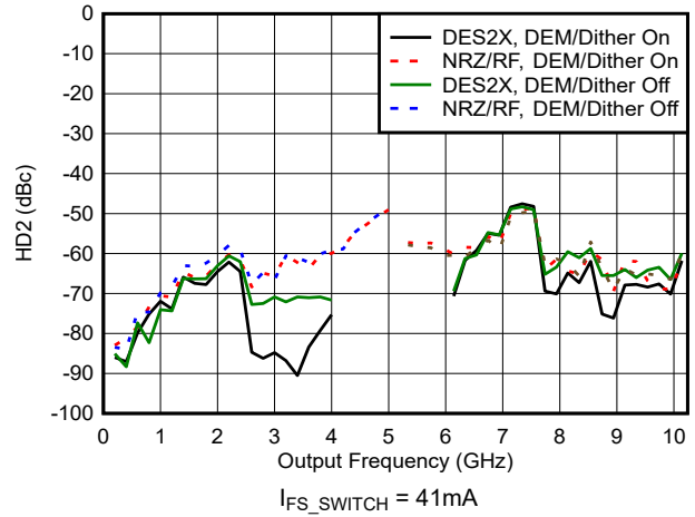
图 6-109. HD2 与频率和模式间的关系
