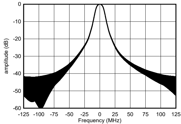
图 9-15. NLFM 线性调频脉冲的数字频谱
