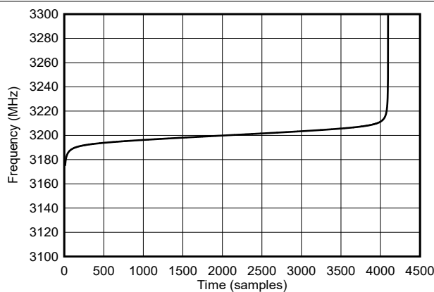
图 9-13. NLFM 频率斜升
