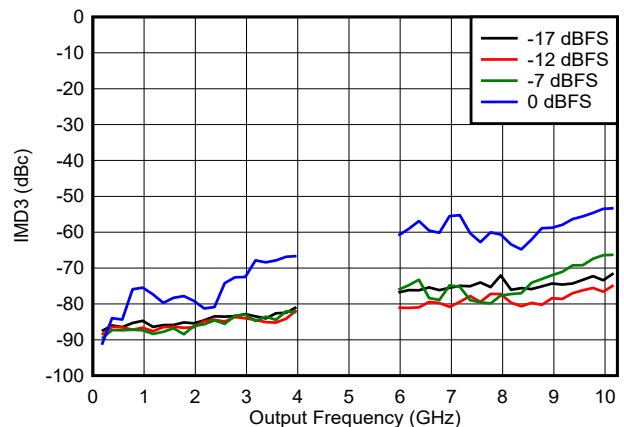
图 6-135. NRZ/RF 模式下 IMD3 与频率和数字振幅间的关系
