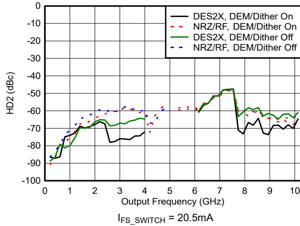
图 6-108. HD2 与频率和模式间的关系
