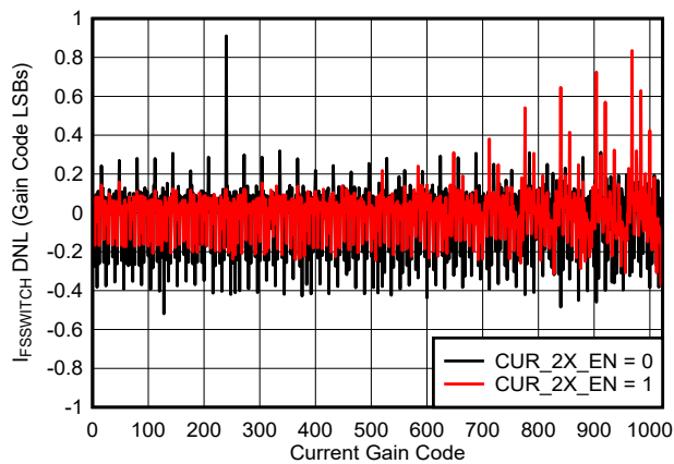
图 6-17. I_{\text{FS\_SWITCH}} 误差与增益代码间的关系
