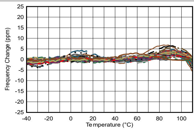
图 6-14. 频率变化与温度间的关系 (25MHz、3.3V 电源电压、80 个器件)
