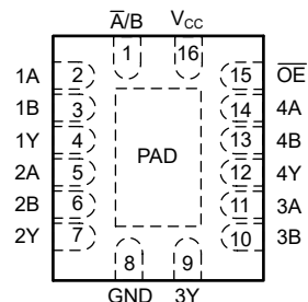
图 3-2. CD74AC257、CD74ACT257、CD74ACT258
