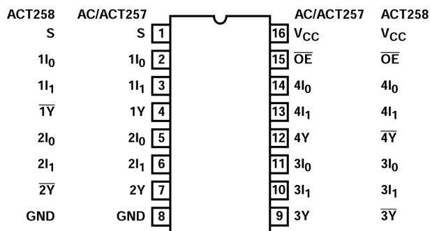
图 3-1. CD54AC257、CD54ACT257 J 封装；
