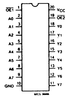
图 3-2. CDx4AC541, CDx4ACT541
