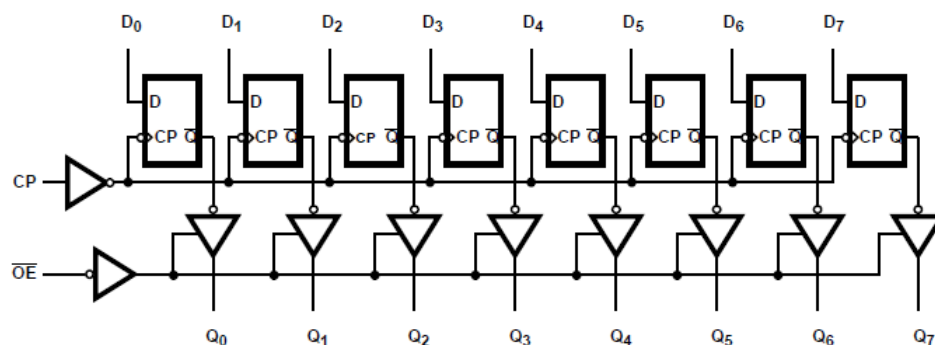
功能图
