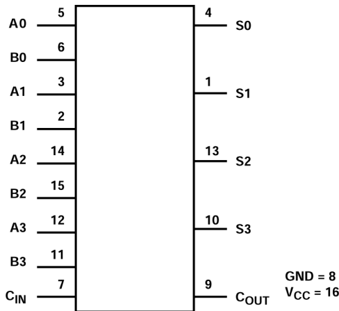
功能方框图
