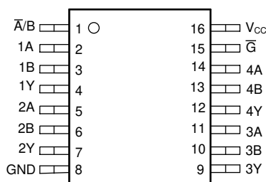
图 4-1. CD54AC157 J 封装 ( 顶视图 )
