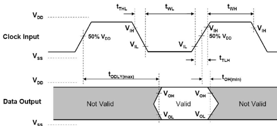
图 6-4. SDIO HS 输出时序
