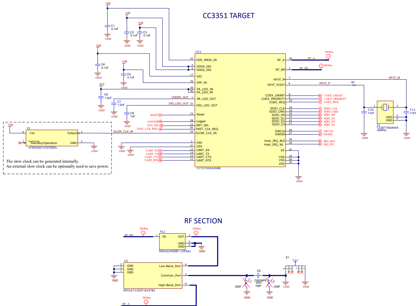
图 8-1. CC335x 参考原理图
