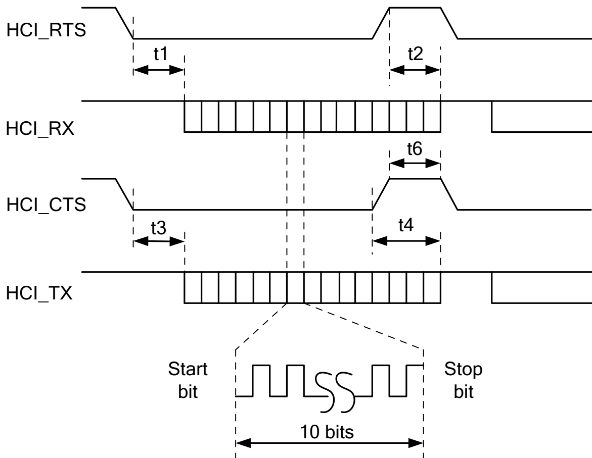
图 6-6. UART 时序图
