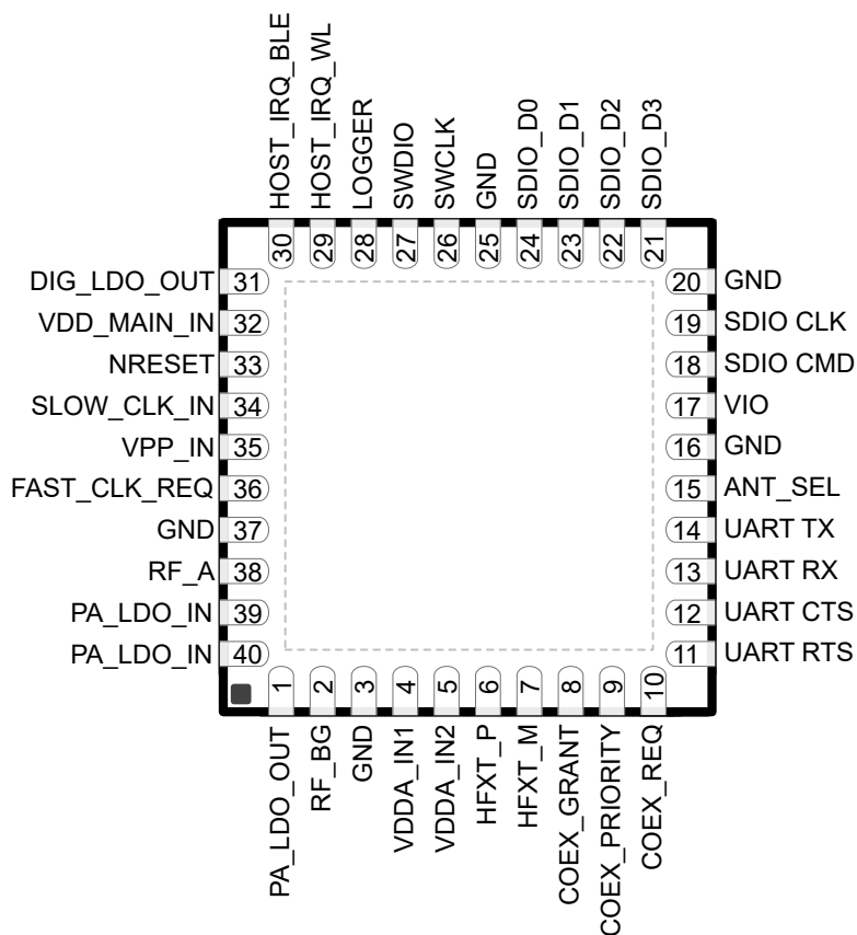
图 5-1. CC3351 引脚图
