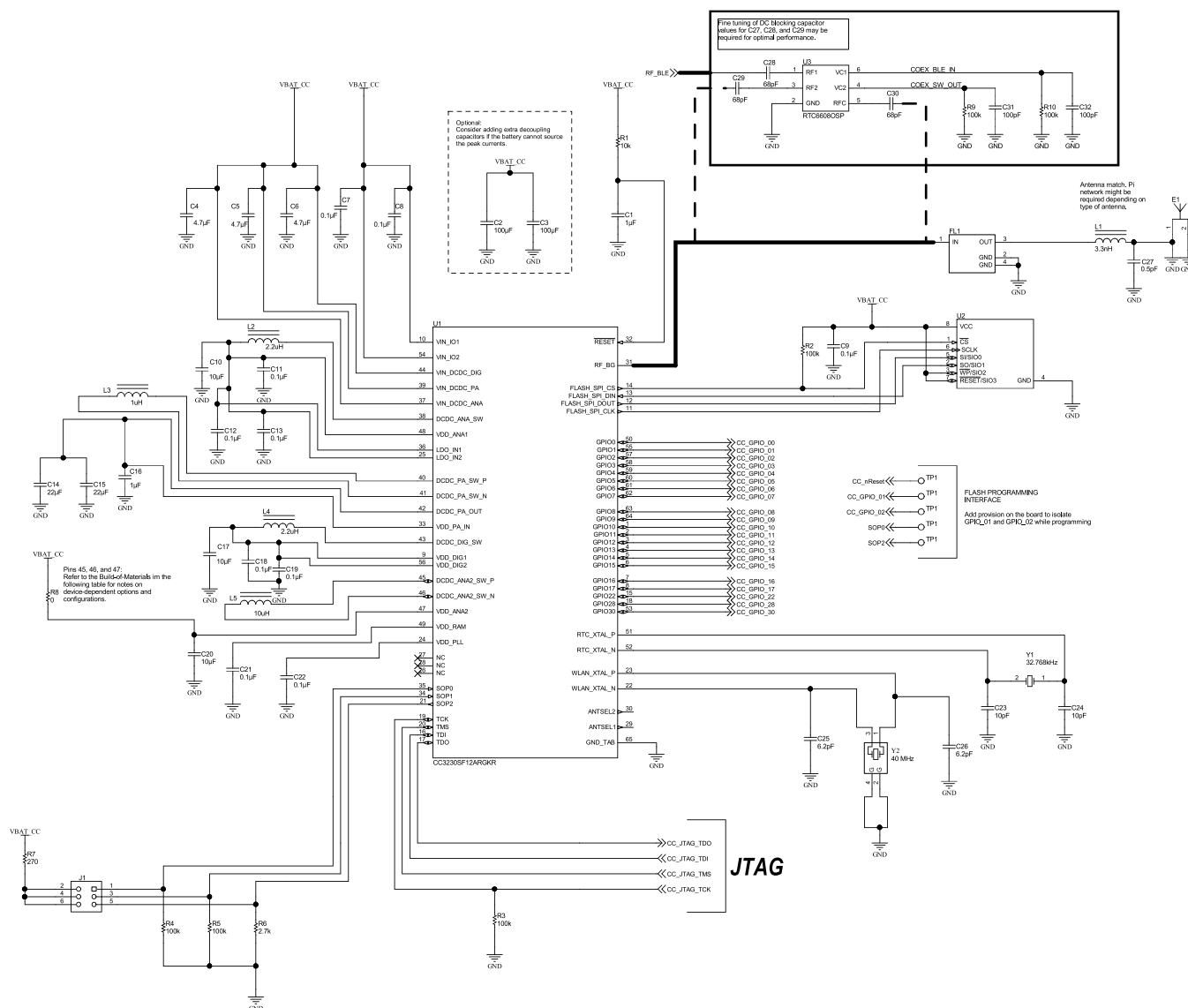
图 9-5. CC3230x Engine Area 和 Optional BLE Coexistence
