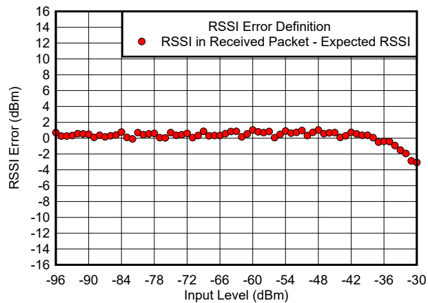
图 7-21. RSSI 误差与输入电平间的关系 (dBm)
