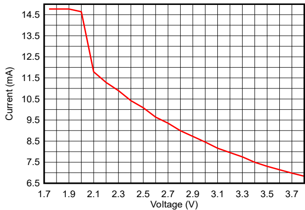
图 7-12. TX 电流与电源电压 (VDD) 间的关系 ( BLE 1Mbps , 2.44GHz , 0dBm )
