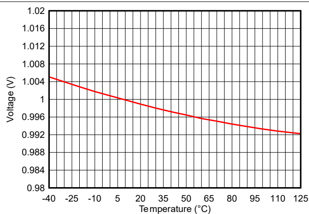
图 7-34. ADC 精度与温度间的关系 ( V_{IN} = 1V , 内部基准, 200ksps)
