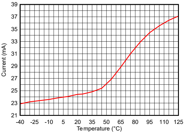
图 7-11. TX 电流与温度间的关系 ( BLE 1Mbps , 2.44GHz , +10dBm ) , VDDS = 3.3V
