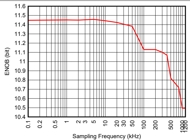
图 7-31. ENOB 与采样频率间的关系 ( V_{in} = 3V 斜坡波, 内部基准, 200ksps )
