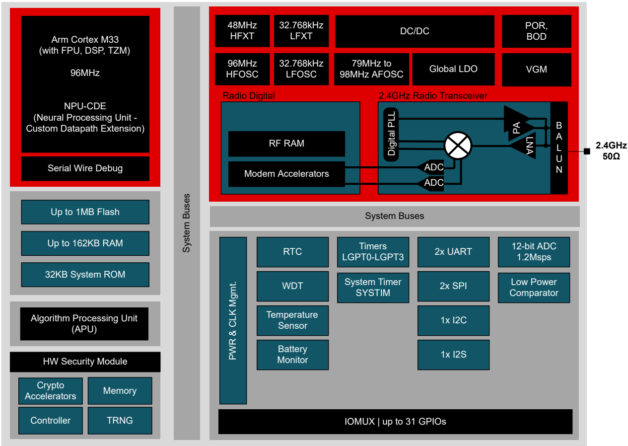
图 4-1. 功能方框图
