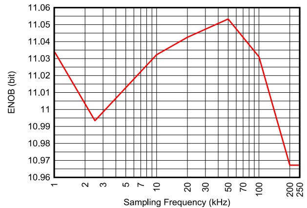
图 7-29. ENOB 与采样频率间的关系 ( V_{in} = 3V 斜坡波, 内部基准, F_{in} = F_s/10 )
