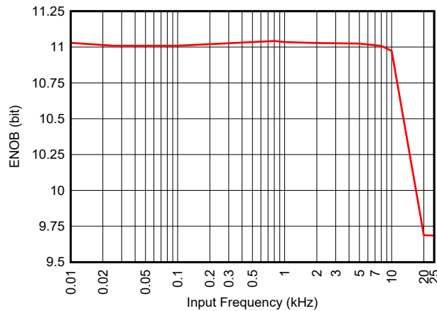
图 7-28. ENOB 与输入频率间的关系 ( 内部基准 )
