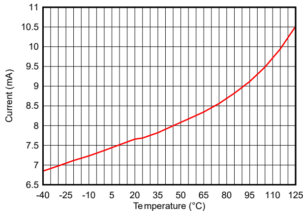
图 7-10. TX 电流与温度间的关系 ( BLE 1Mbps , 2.44GHz , 0dBm ) , VDDS = 3.3V
