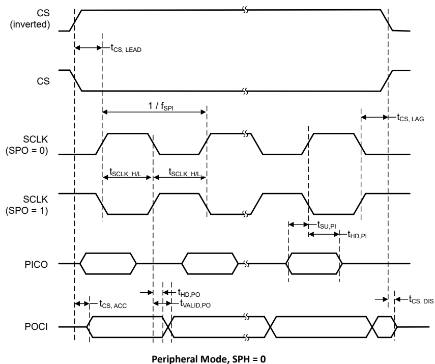
图 7-3. SPI 计时示意图 - 外设模式，SPH = 0
