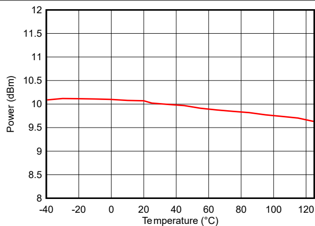
图 7-23. 输出功率与温度间的关系 ( BLE 1Mbps , 2.44GHz , +10dBm )
