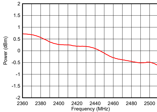
图 7-26. 输出功率与频率间的关系 ( BLE 1Mbps , 0dBm )
