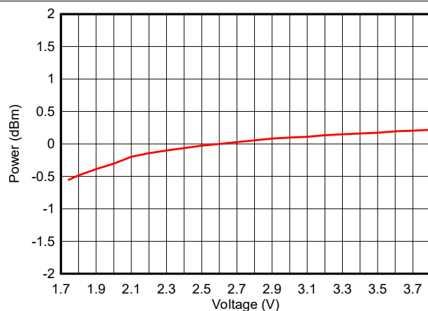
图 7-24. 输出功率与电源电压 (VDD) 间的关系 ( BLE 1Mbps , 2.44GHz , 0dBm )
