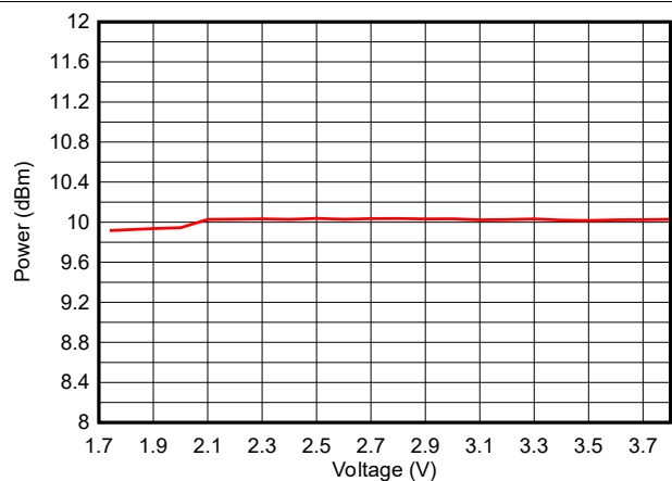
图 7-25. 输出功率与电源电压 (VDD) 间的关系 ( BLE 1Mbps , 2.44GHz , +10dBm )
