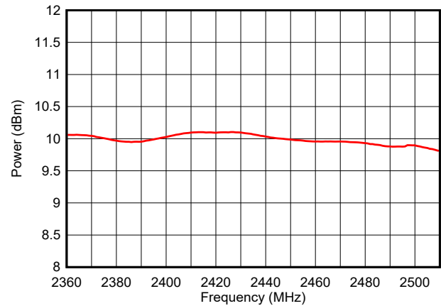
图 7-27. 输出功率与频率间的关系 ( BLE 1Mbps , +10dBm )
