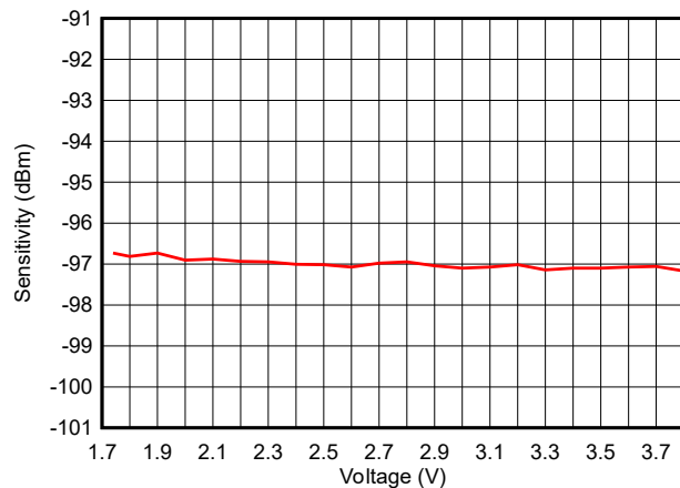
图 7-20. 灵敏度与电源电压 (VDD) 间的关系 ( BLE 1Mbps , 2.44GHz , 禁用直流/直流转换器 )
