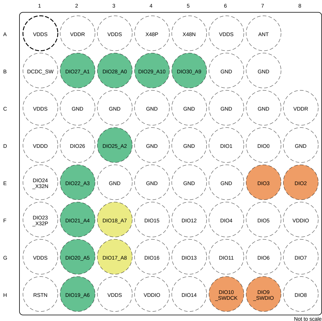
图 6-2. YCJ WCSP 引脚排列 (顶视图)
