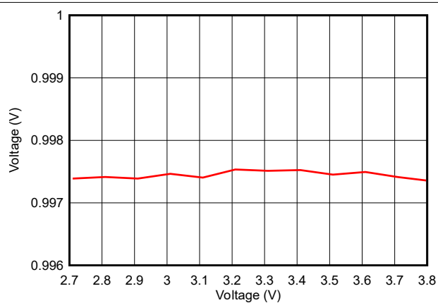
图 7-35. ADC 精度与电源电压间的关系 ( V_{IN} = 1V , 内部基准, 200ksps)
