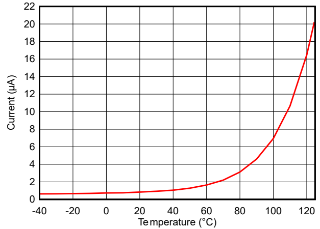
图 7-7. 待机模式 (MCU) 电流与温度间的关系 (SRAM 和部分寄存器保留, 启用 RTC), V_{DD5} = 3.3\text{V}
