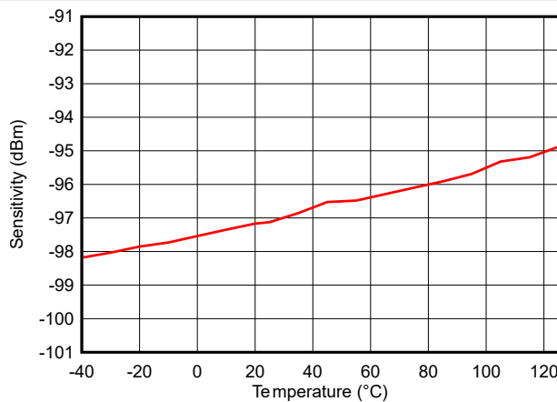
图 7-16. 灵敏度与温度间的关系 ( BLE 1Mbps , 2.44GHz )
