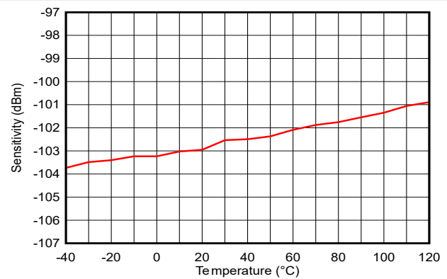
图 7-17. 灵敏度与温度间的关系 (IEEE 802.15.4 PHY)
