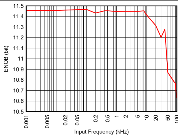
图 7-30. ENOB 与输入频率间的关系 ( 外部基准 = 3.0V )
