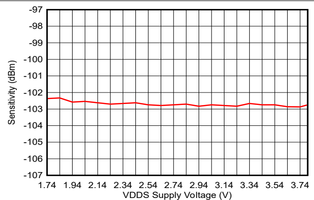
图 7-19. 灵敏度与 VDDDS 间的关系 (IEEE 802.15.4 PHY)
