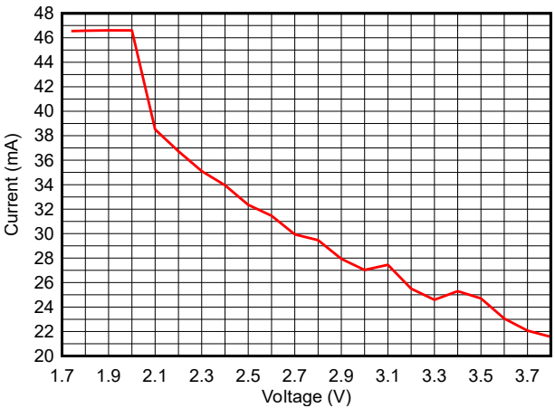
图 7-13. TX 电流与电源电压 (VDD) 间的关系 ( BLE 1Mbps , 2.44GHz , +10dBm )
