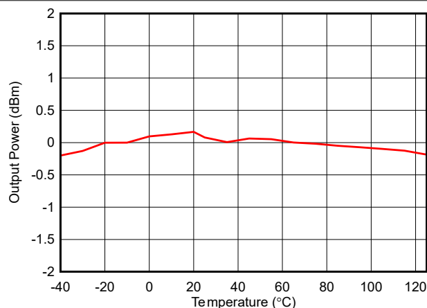
图 7-22. 输出功率与温度间的关系 ( BLE 1Mbps , 2.44GHz , 0dBm )
