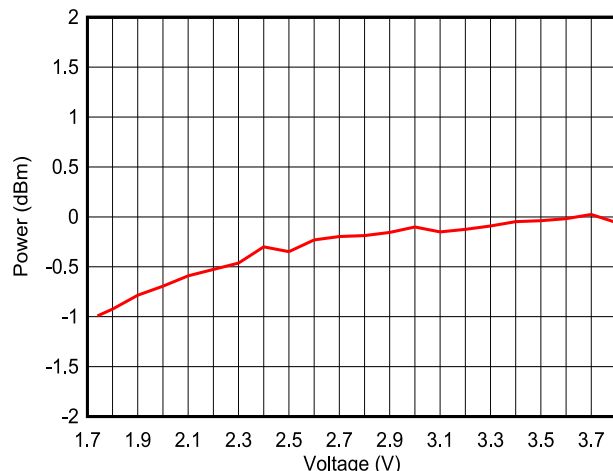
图 7-24. 输出功率与电源电压 (VDD5) 间的关系 (LE 1M PHY, 2.44GHz, 0dBm)
