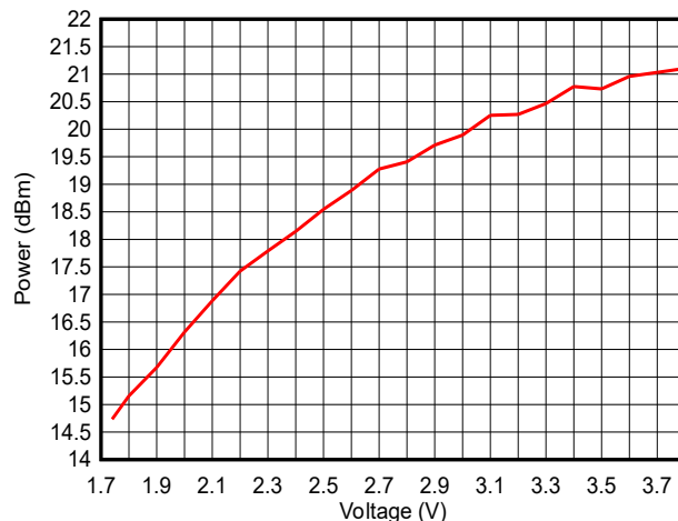
图 7-25. 输出功率与电源电压 (VDD5) 间的关系 (LE 1M PHY, 2.44GHz, +20dBm)
