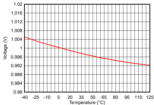
图 7-34. ADC 精度与温度间的关系 ( V_{IN} = 1V , 内部基准, 200ksps )
