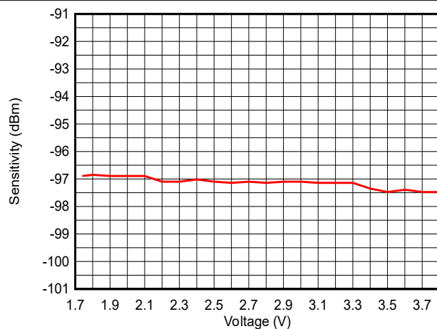
图 7-18. 灵敏度与电源电压 (VDDDS) 间的关系 (LE 1M PHY , 2.44GHz)
