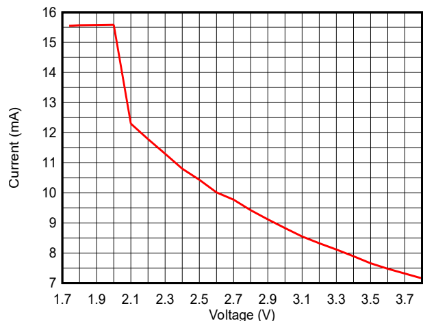
图 7-12. TX 电流与电源电压 (VDD5) 间的关系 ( LE 1M PHY , 2.44GHz , 0dBm )
