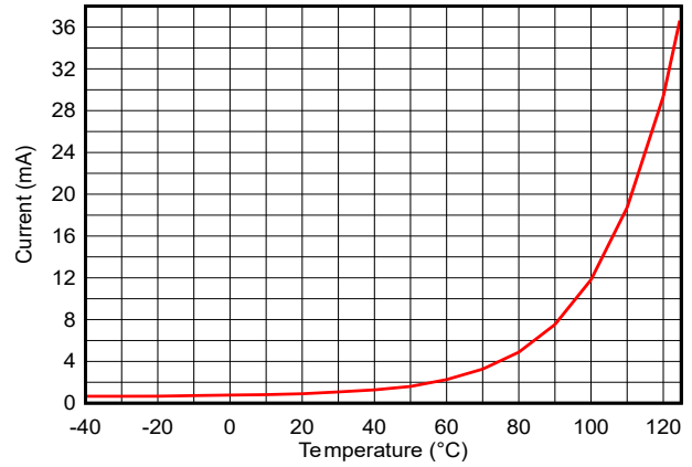
图 7-7. 待机模式 (MCU) 电流与温度间的关系 (SRAM 和部分寄存器保留, 启用 RTC), V_{DD5} = 3.3\text{V}
