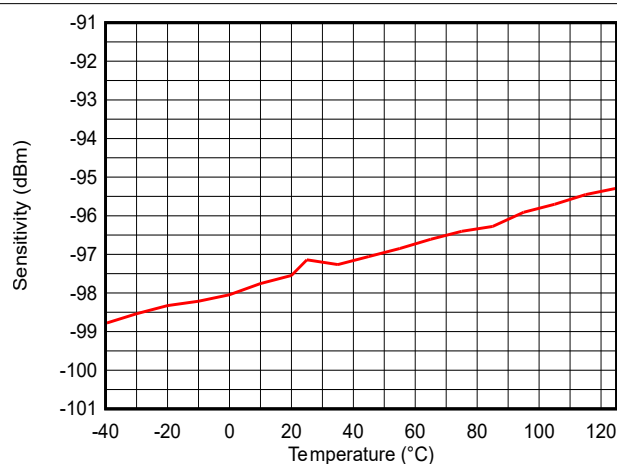
图 7-16. 灵敏度与温度间的关系 (LE 1M PHY , 2.44GHz)
