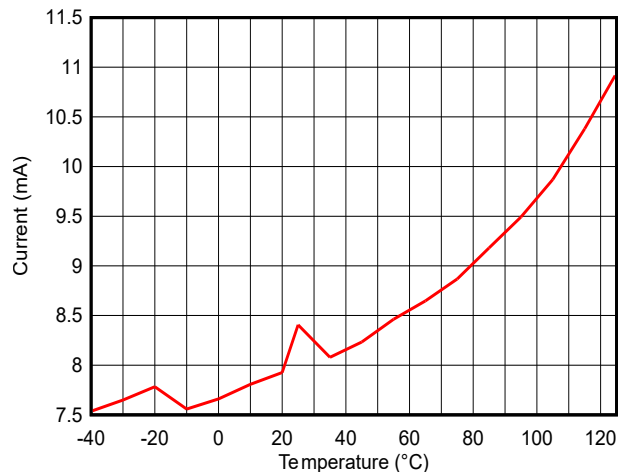
图 7-10. TX 电流与温度间的关系 ( LE 1M PHY , 2.44GHz , 0dBm ) , VDD5 = 3.3V
