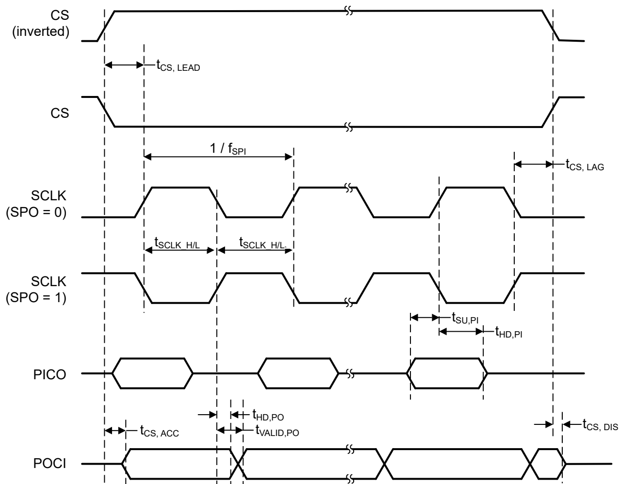
图 7-3. SPI 计时示意图 - 外设模式, SPH = 0
