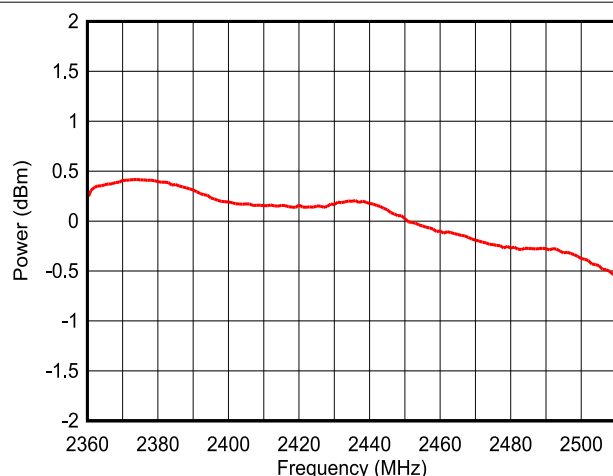
图 7-26. 输出功率与频率间的关系 (LE 1M PHY, 0dBm)
