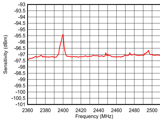
图 7-14. 灵敏度与频率间的关系 (LE 1M PHY)
