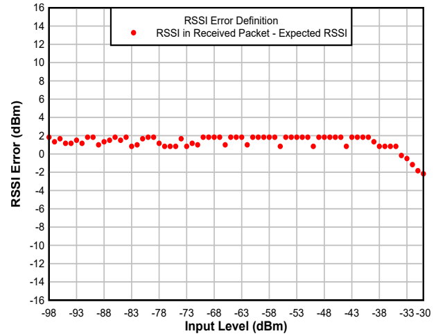
图 7-21. RSSI 误差与输入电平间的关系 (dBm)
