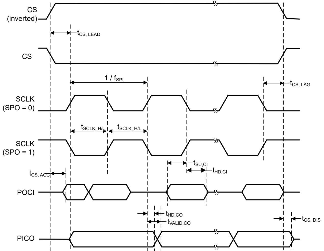
图 7-2. SPI 计时示意图 - 控制器模式, SPH = 1
