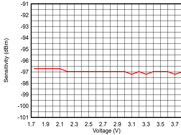
图 7-20. 灵敏度与电源电压 (VDD SS ) 间的关系 (LE 1M PHY, 2.44GHz, 禁用直流/直流转换器)
