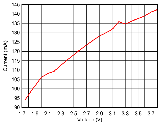
图 7-13. TX 电流与电源电压 (VDD5) 间的关系 ( LE 1M PHY , 2.44GHz , +20dBm )
