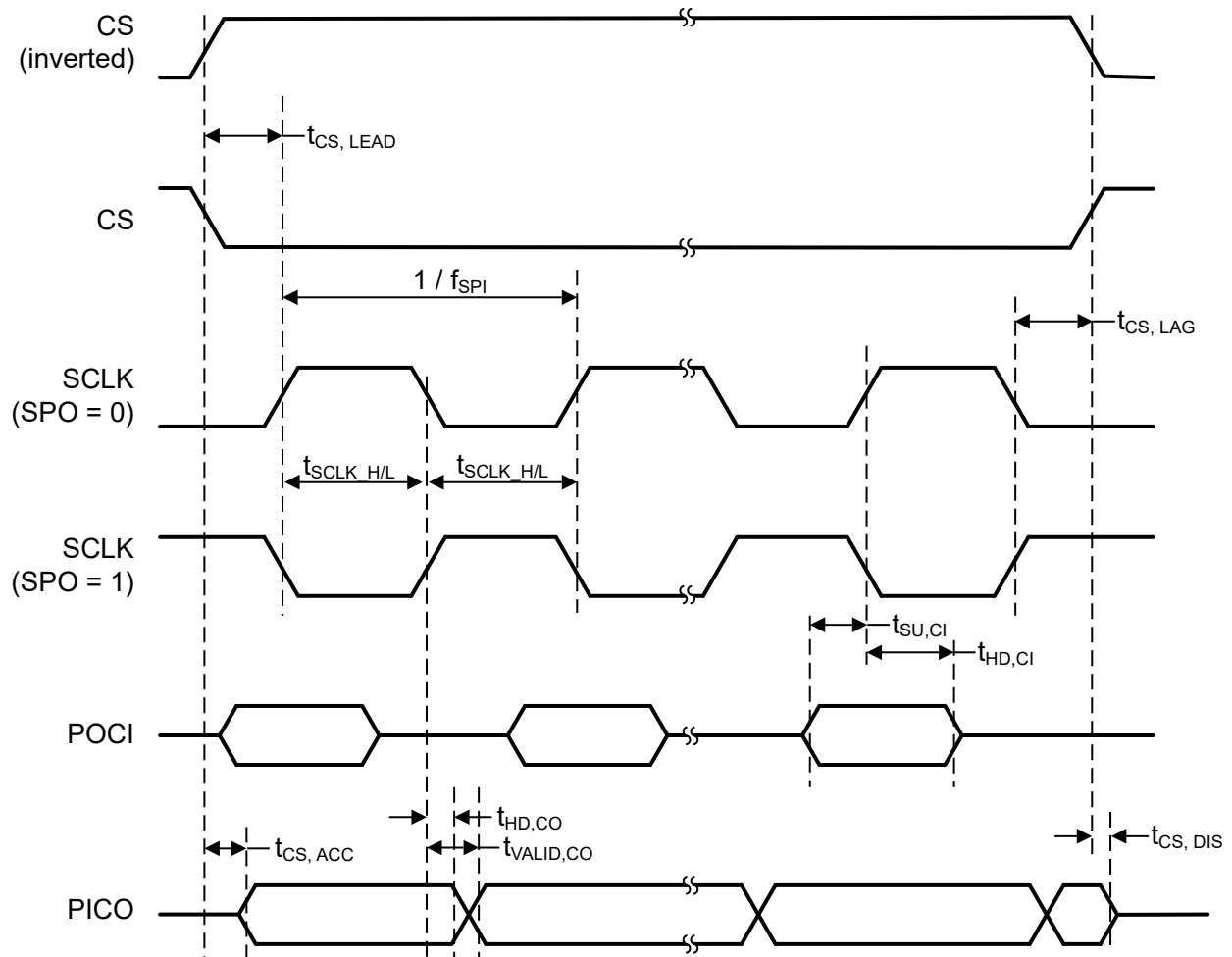
图 7-1. SPI 计时示意图 - 控制器模式, SPH = 0
