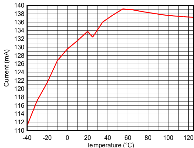
图 7-11. TX 电流与温度间的关系 ( LE 1M PHY , 2.44GHz , +20dBm ) , VDD5 = 3.3V
