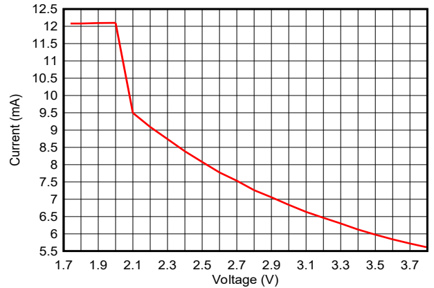
图 7-9. RX 电流与电源电压 ( V_{DD5} ) 间的关系 (LE 1M PHY, 2.44GHz)
