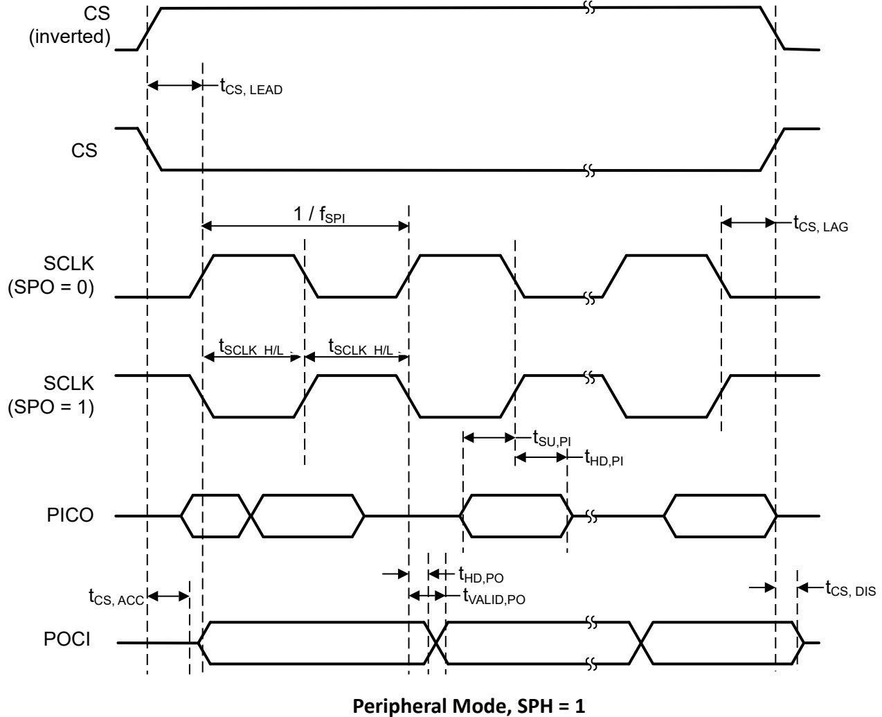
图 7-4. SPI 计时示意图 - 外设模式，SPH = 1
