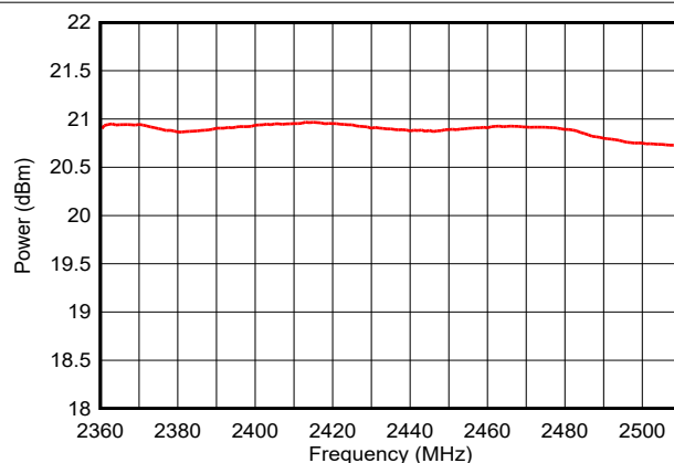
图 7-27. 输出功率与频率间的关系 (LE 1M PHY, +20dBm)
