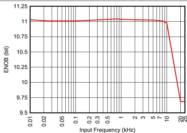
图 7-28. ENOB 与输入频率间的关系 (内部基准)
