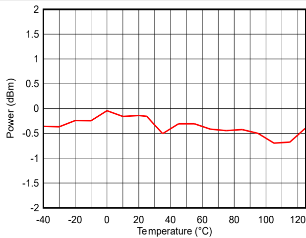
图 7-22. 输出功率与温度间的关系 (LE 1M PHY, 2.44GHz, 0dBm)
