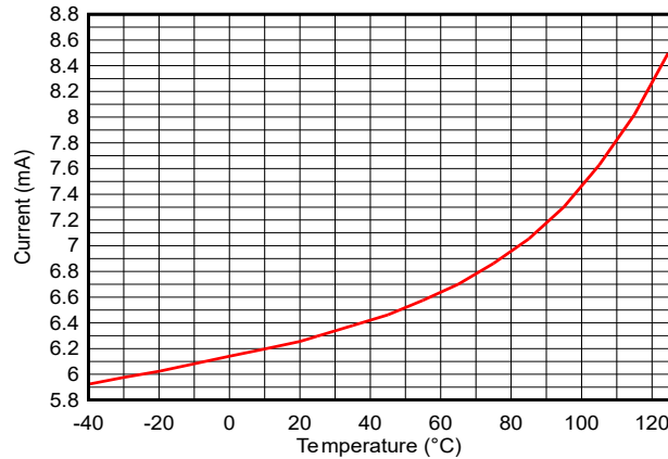
图 7-8. RX 电流与温度间的关系 (LE 1M PHY, 2.44GHz), V_{DD5} = 3.3\text{V}
