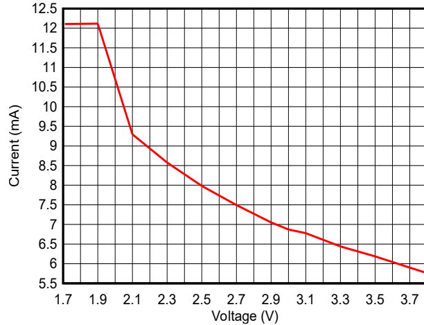
图 7-6. 工作模式 (MCU) 电流与电源电压 ( V_{DD5} ) 间的关系 (运行 CoreMark)
