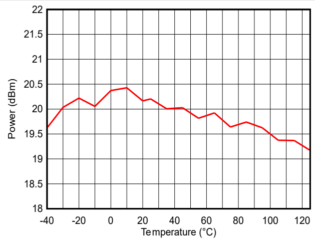
图 7-23. 输出功率与温度间的关系 (LE 1M PHY, 2.44GHz, +20dBm)
