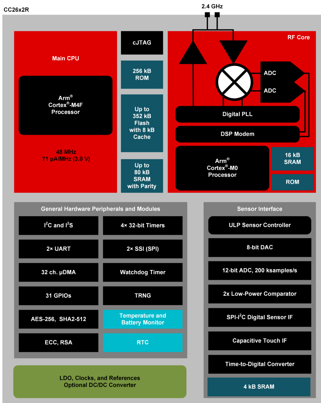
图 4-1. CC2652R 方框图
