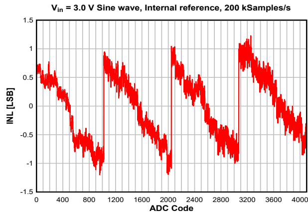
图 8-25. INL vs. ADC Code
