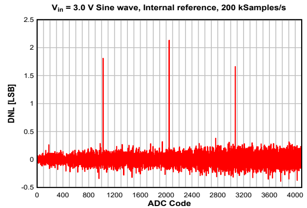
图 8-26. DNL vs. ADC Code
