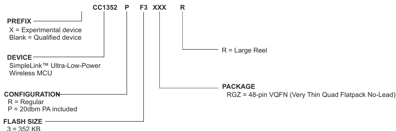
图 11-1. Device Nomenclature
