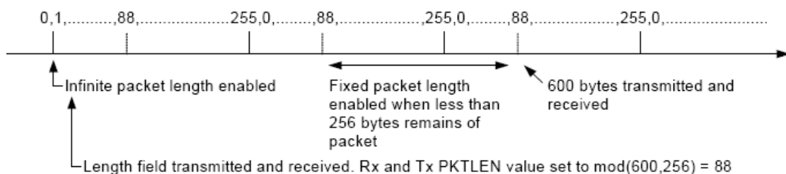
图 16 数据包长度>255
