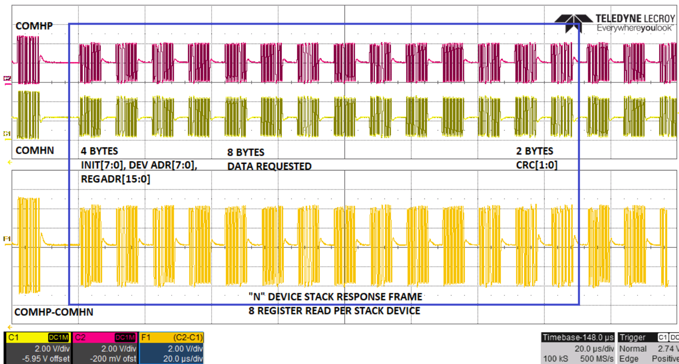
图 8-10. 从堆栈器件读取 8 个寄存器的响应帧
