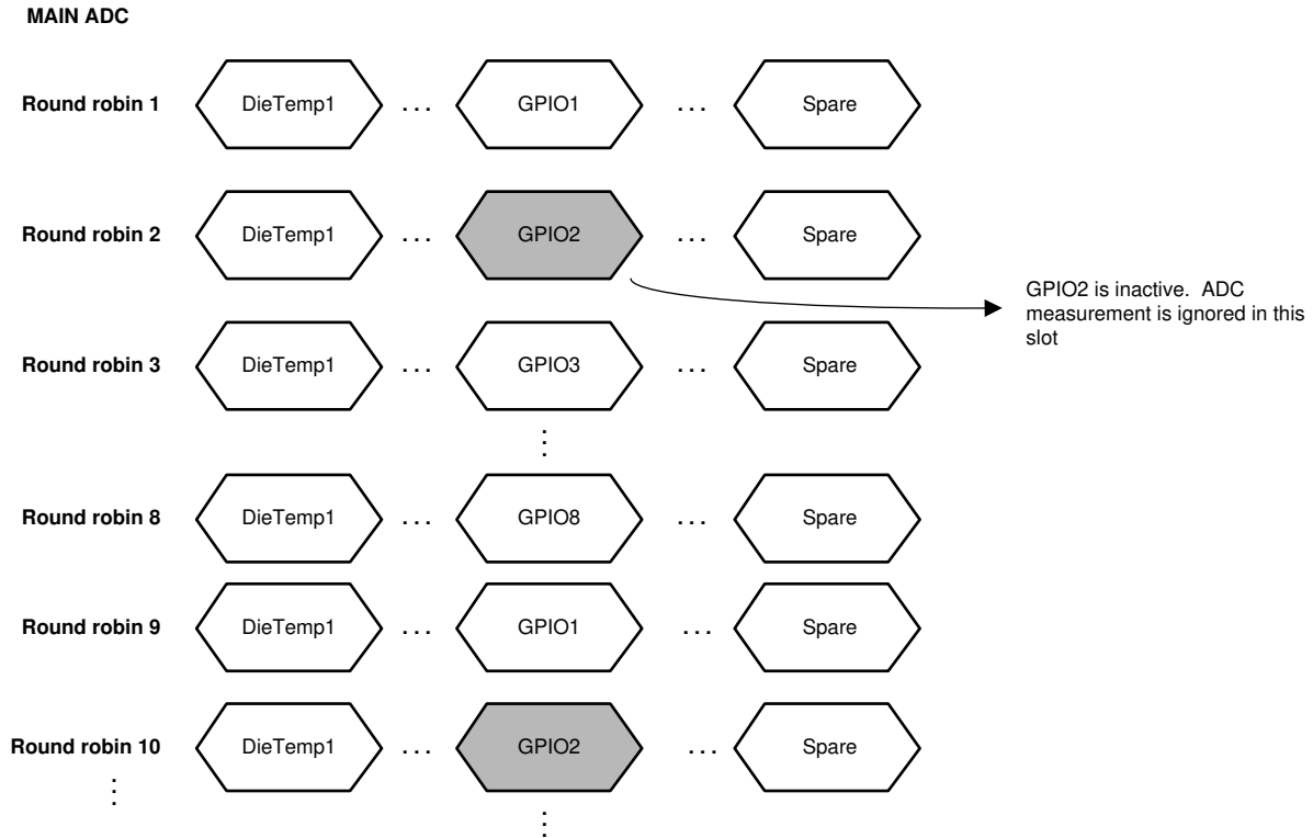
图 7-7. GPIO2 未配置用于 ADC 测量
