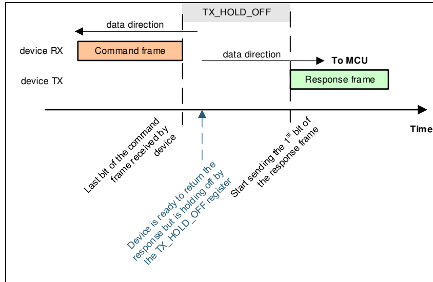
图 7-25. UART TX_HOLD_OFF
