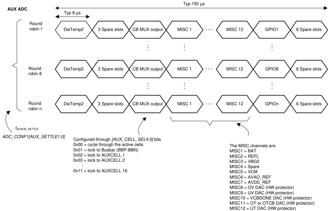
图 7-9. AUX ADC 轮询测量
