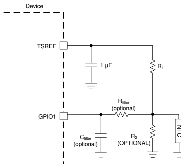
图 7-6. 热敏电阻连接
