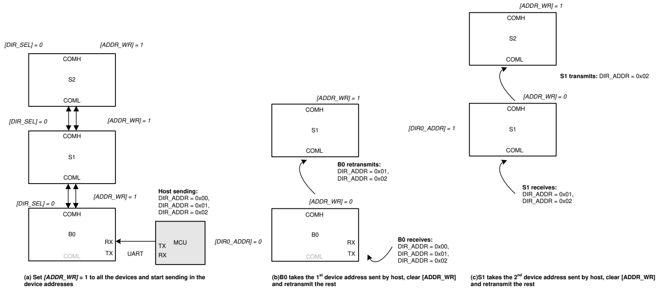
图 7-36. 自动寻址
