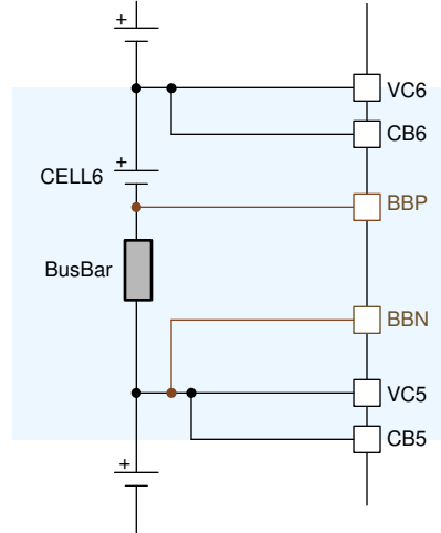
图 7-5. 简化的 BBP 和 BBN 连接
