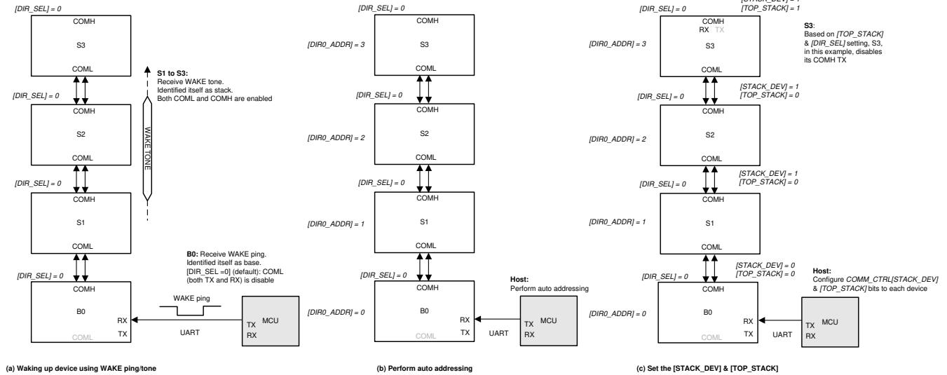
图 7-35. 配置器件进行通信
