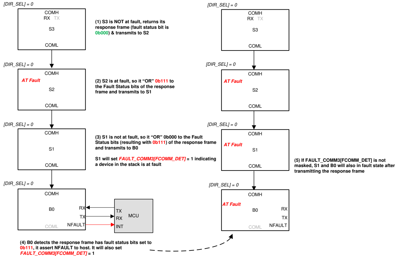
图 7-43. ACTIVE 模式下的传输故障状态 (响应单器件读取)
