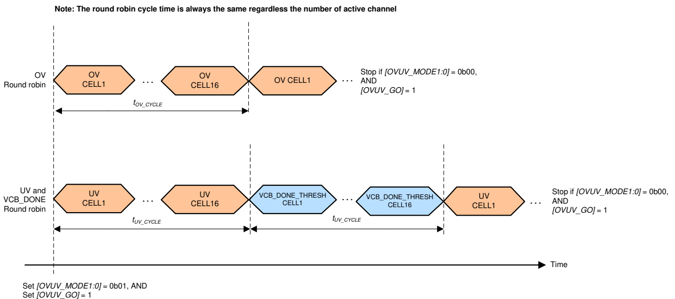
图 7-20. OV 和 UV 轮询模式
