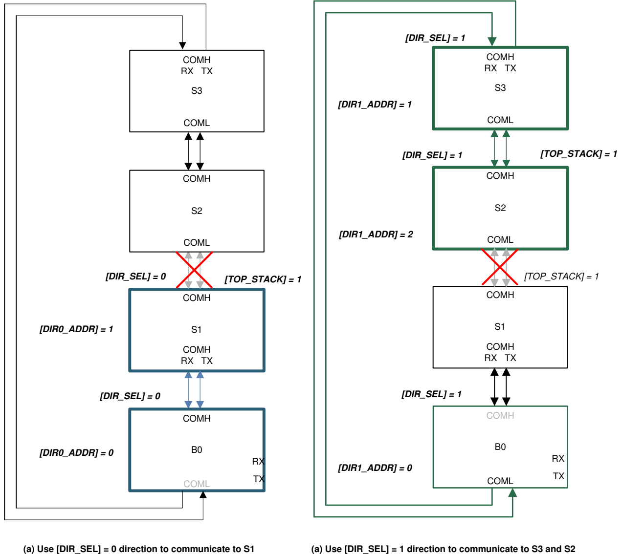
图 7-38. 使用环形架构在电缆断开的情况下访问所有器件
