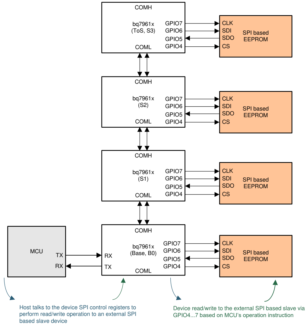
图 7-39. SPI 主器件堆栈配置
