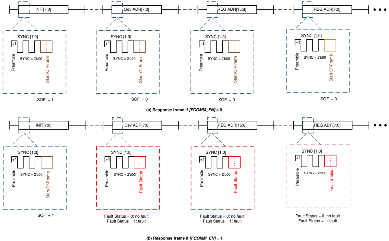
图 7-42. 在通信响应帧中嵌入故障状态
