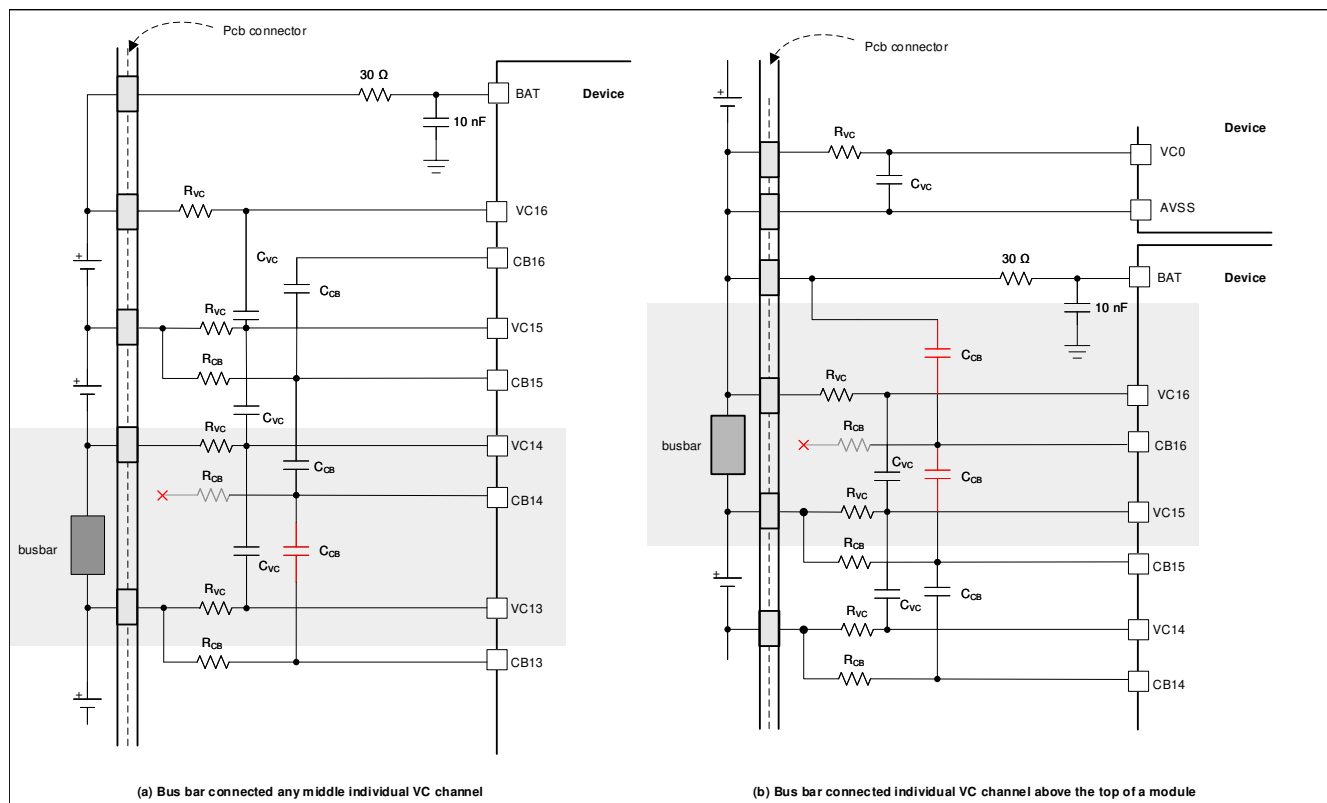
图 7-56. 连接到单个 VC 通道的汇流条
