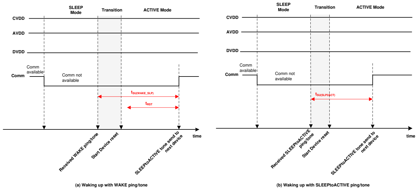
图 7-61. SLEEP 至 ACTIVE 模式转换
