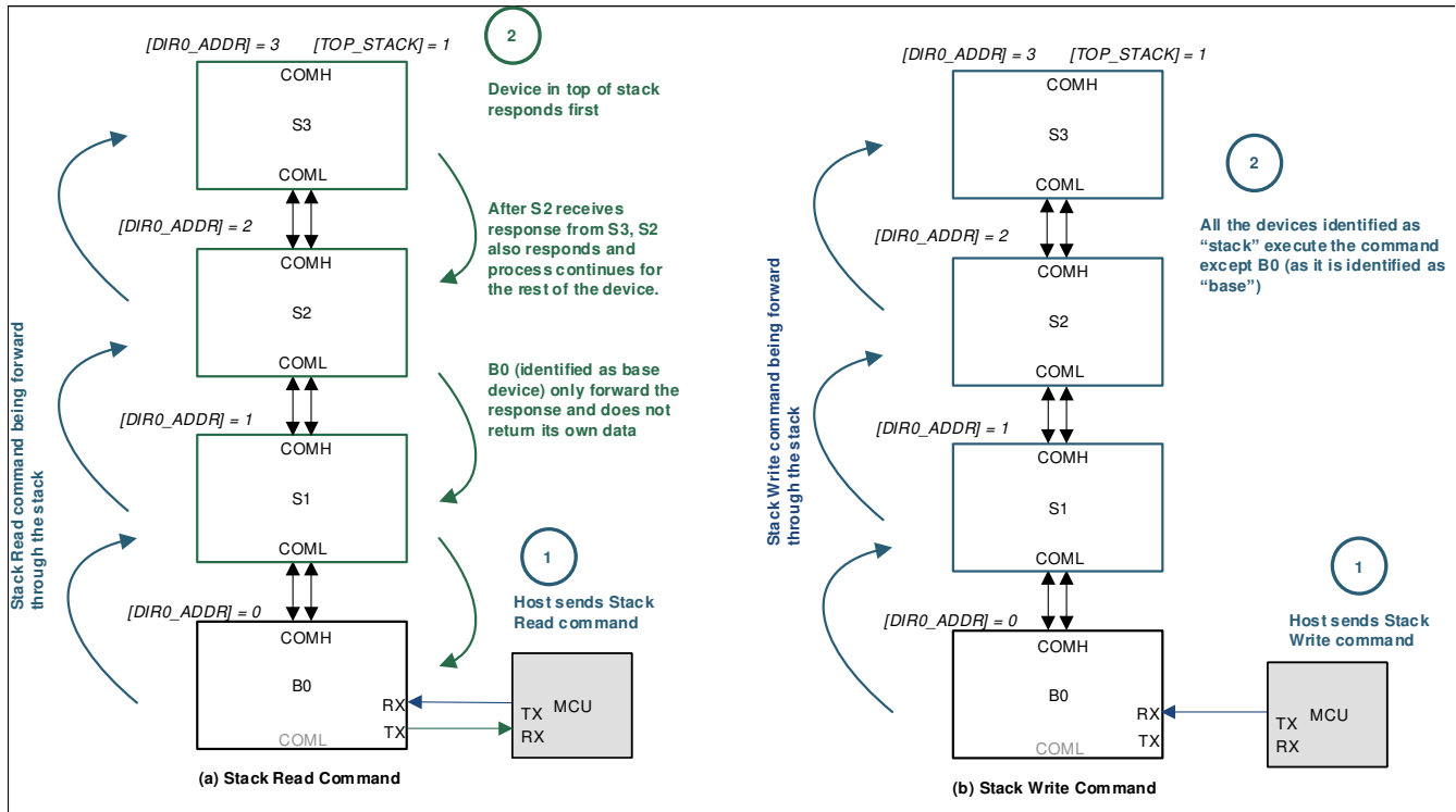
图 7-29. 堆栈读取/写入
