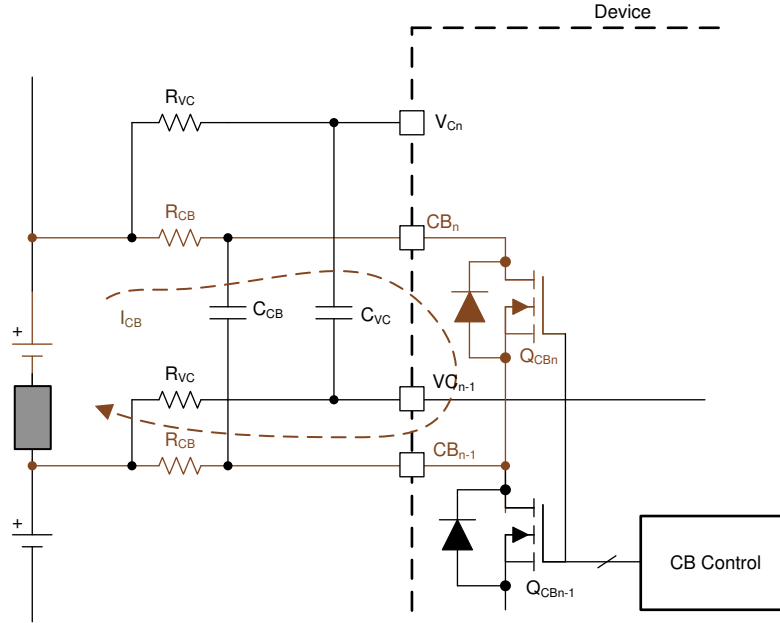
图 7-53. 通过共享电芯通道的汇流条 (通过 BBP/N) 进行电芯均衡
