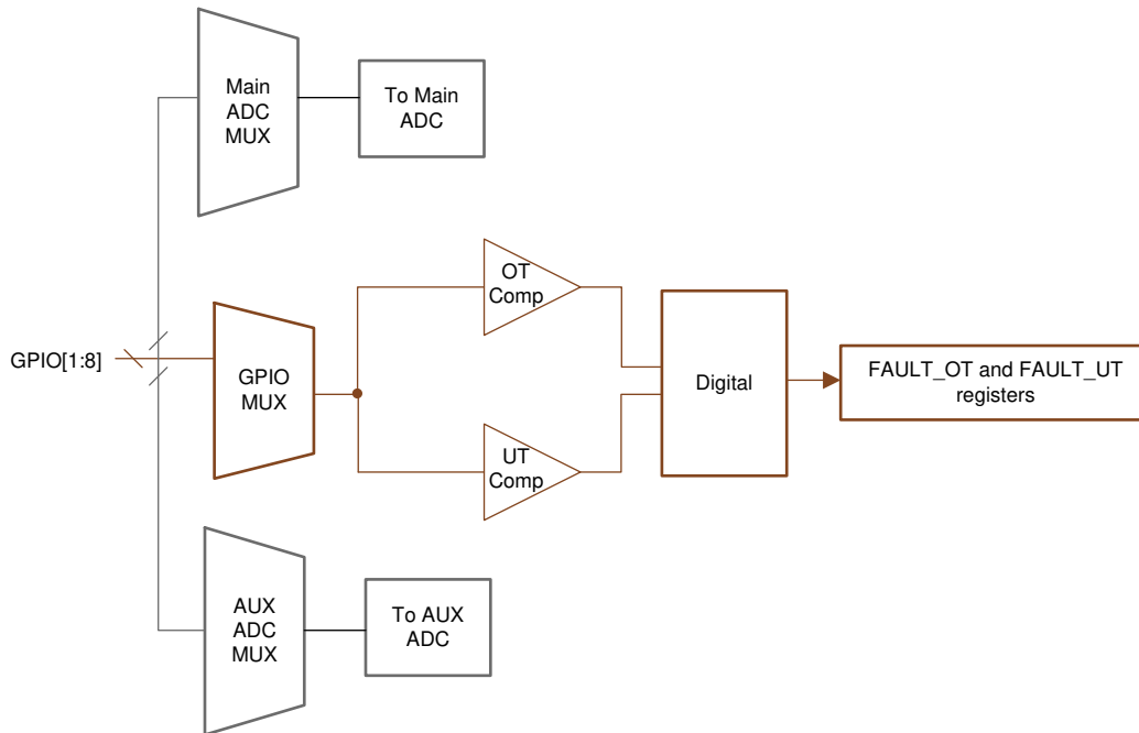
图 7-21. OT 和 UT 保护器
