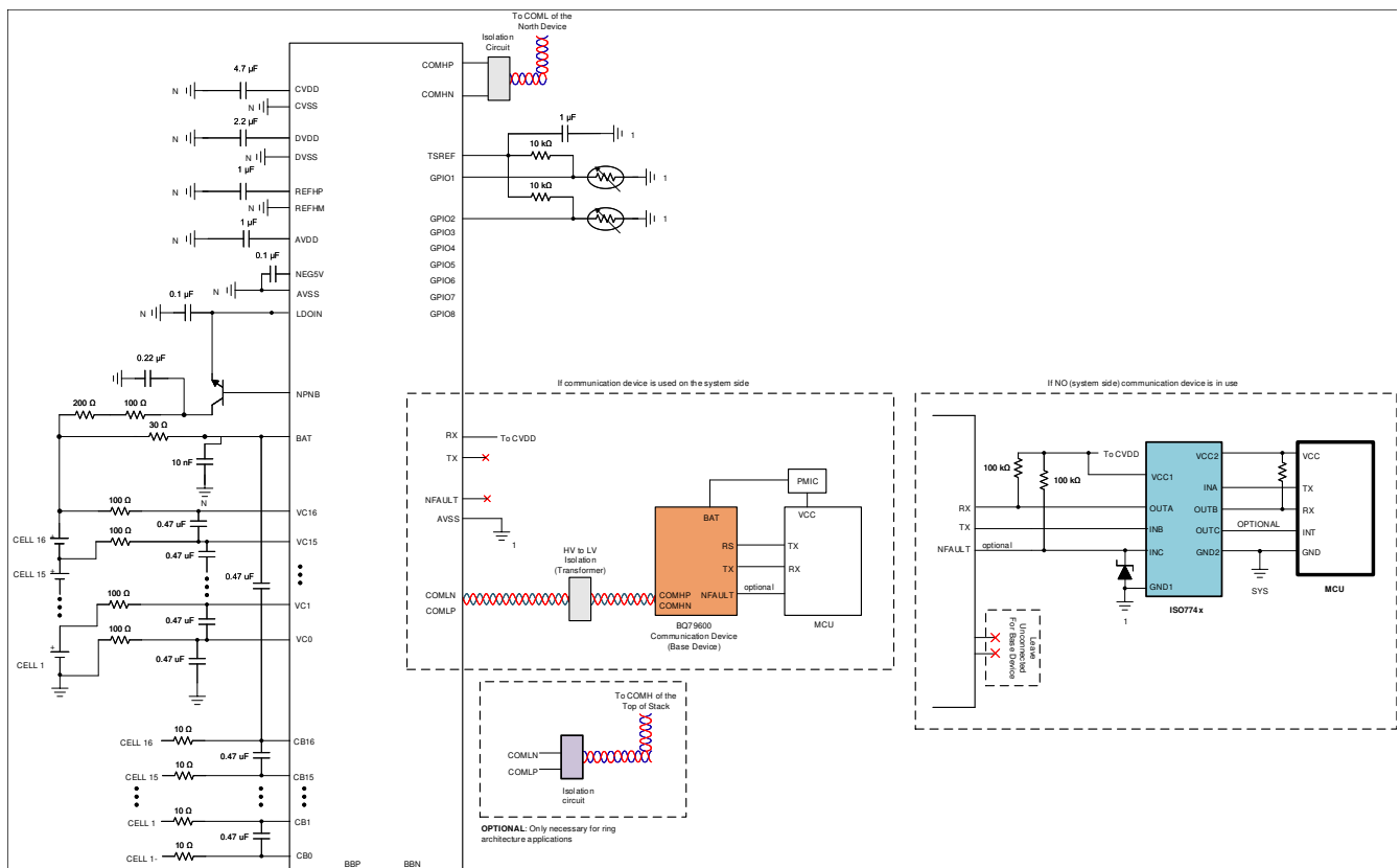
图 8-1. 具有测量应用电路的典型基底器件
