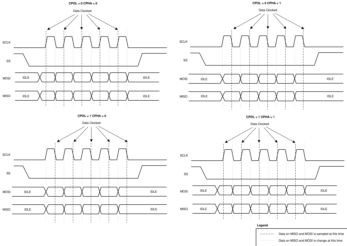
图 7-40. SPI 主器件 CPOL 和 CPHA
