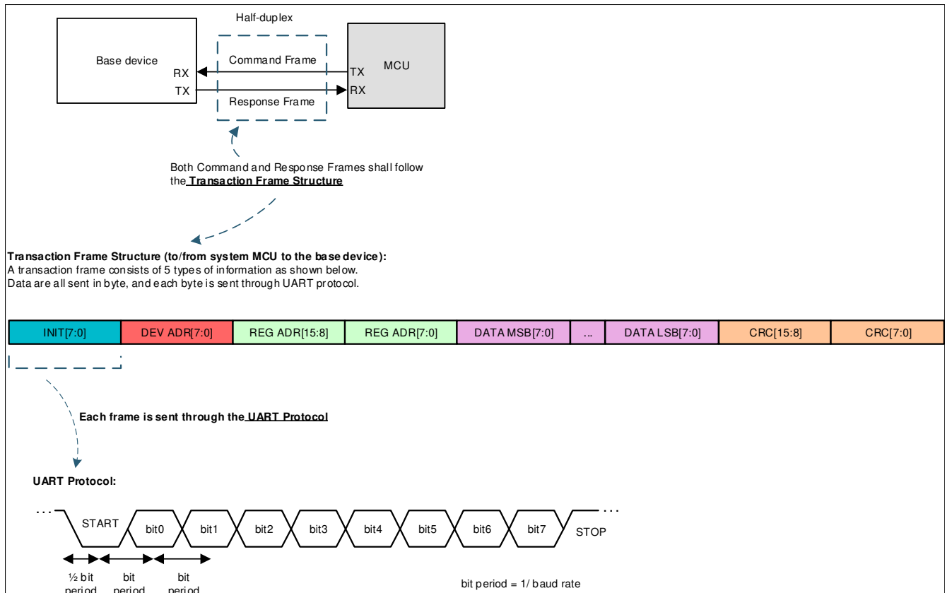
图 7-23. 与主机的 UART 通信
