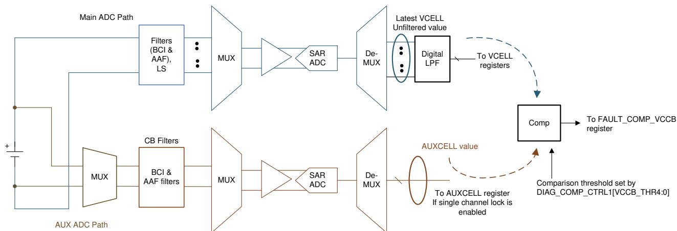
图 7-47. 电芯电压测量诊断
