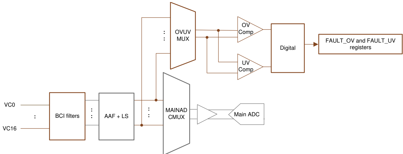
图 7-19. OV 和 UV 保护器
