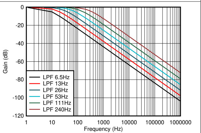
图 6-4. 数字低通滤波器
