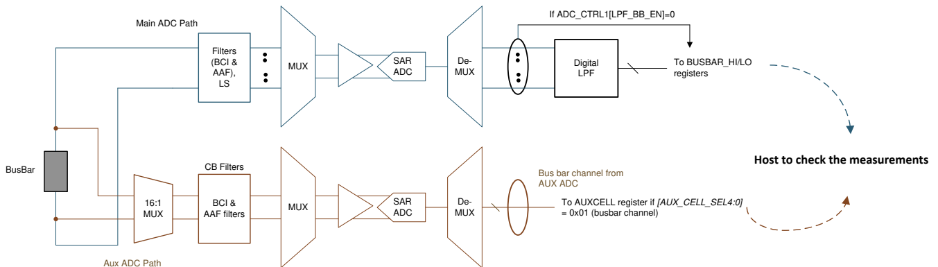
图 7-54. 通过 BBP/N 的汇流条测量检查
