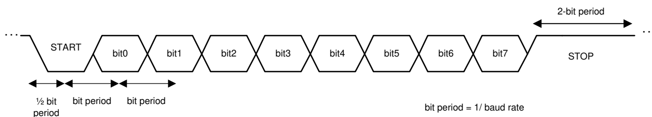
图 7-24. 具有两个 STOP 位的 UART 响应帧
