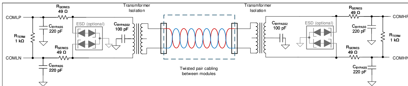
图 8-9. 变压器隔离
