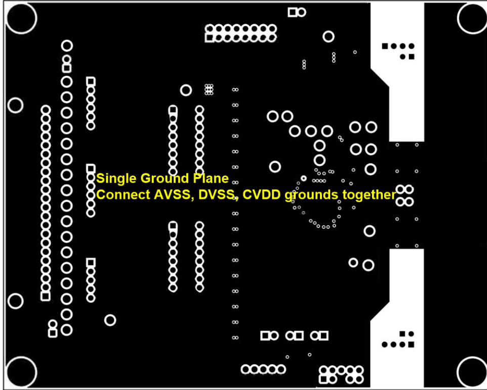
图 10-6. 具有单个接地平面的第三层
