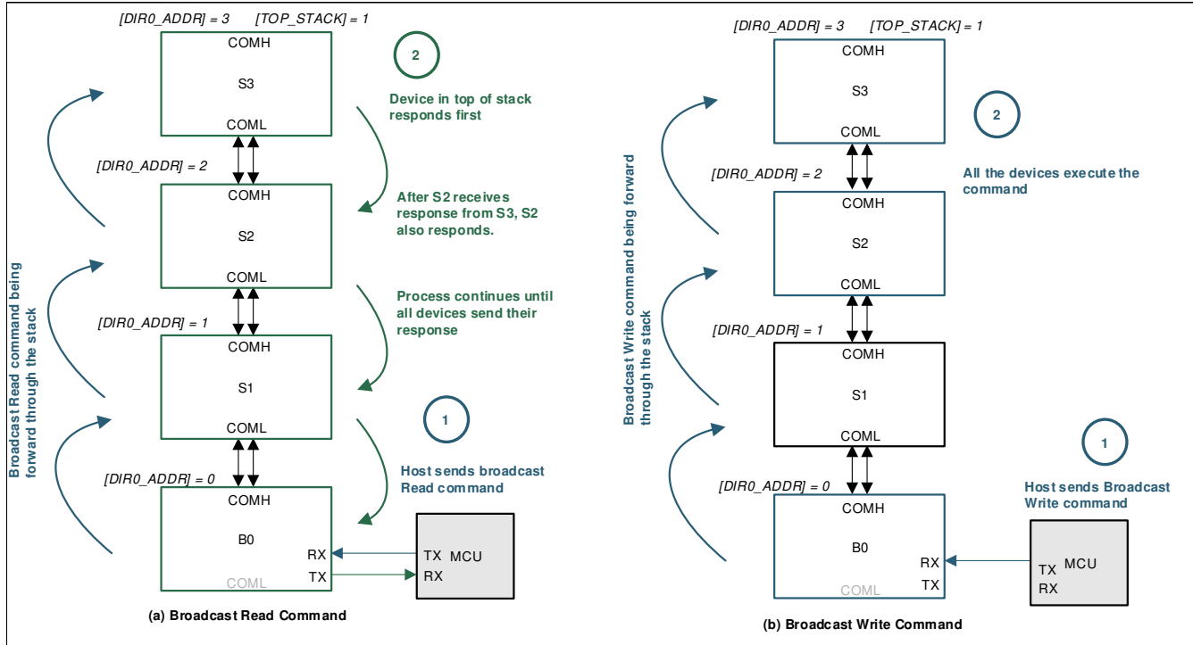
图 7-30. 广播读取/写入
