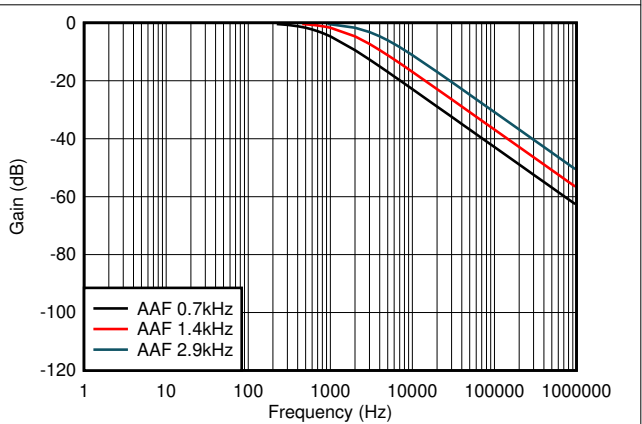
图 6-6. AUX ADC 滤波器
