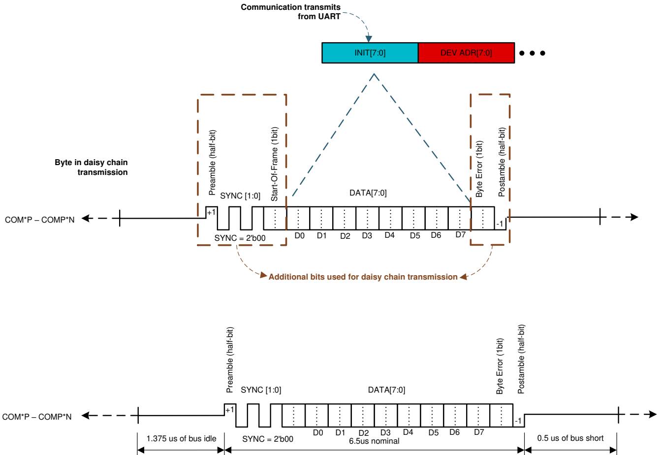
图 7-33. 菊花链字节定义
