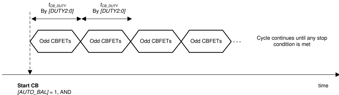
图 7-15. 自动均衡控制，示例 2
