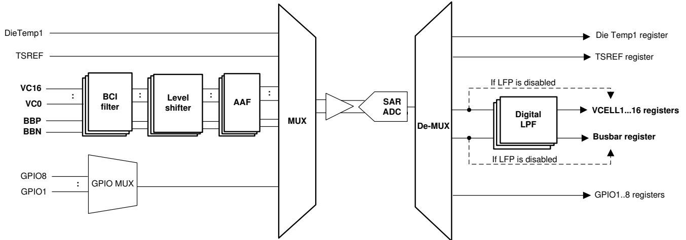
图 7-2. 主 ADC 测量路径
