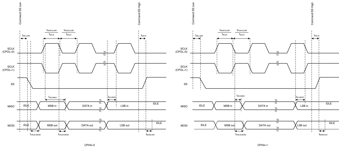
图 7-41. SPI 主器件时序图
