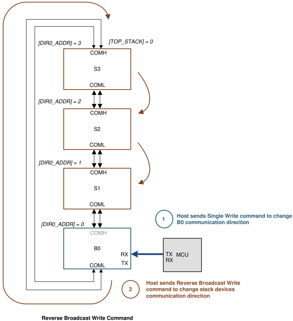
图 7-31. 广播写入反向
