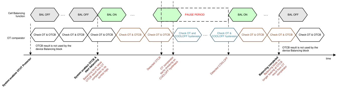
图 7-17. 通过 OTCB 检测暂停和恢复电芯均衡
