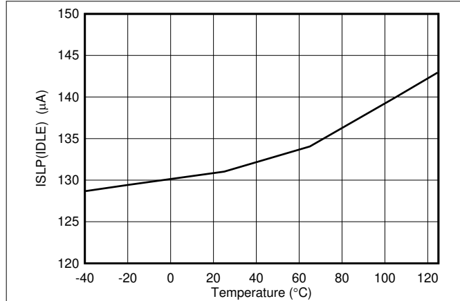
图 6-1. ISLP (IDLE) 与温度之间的关系
