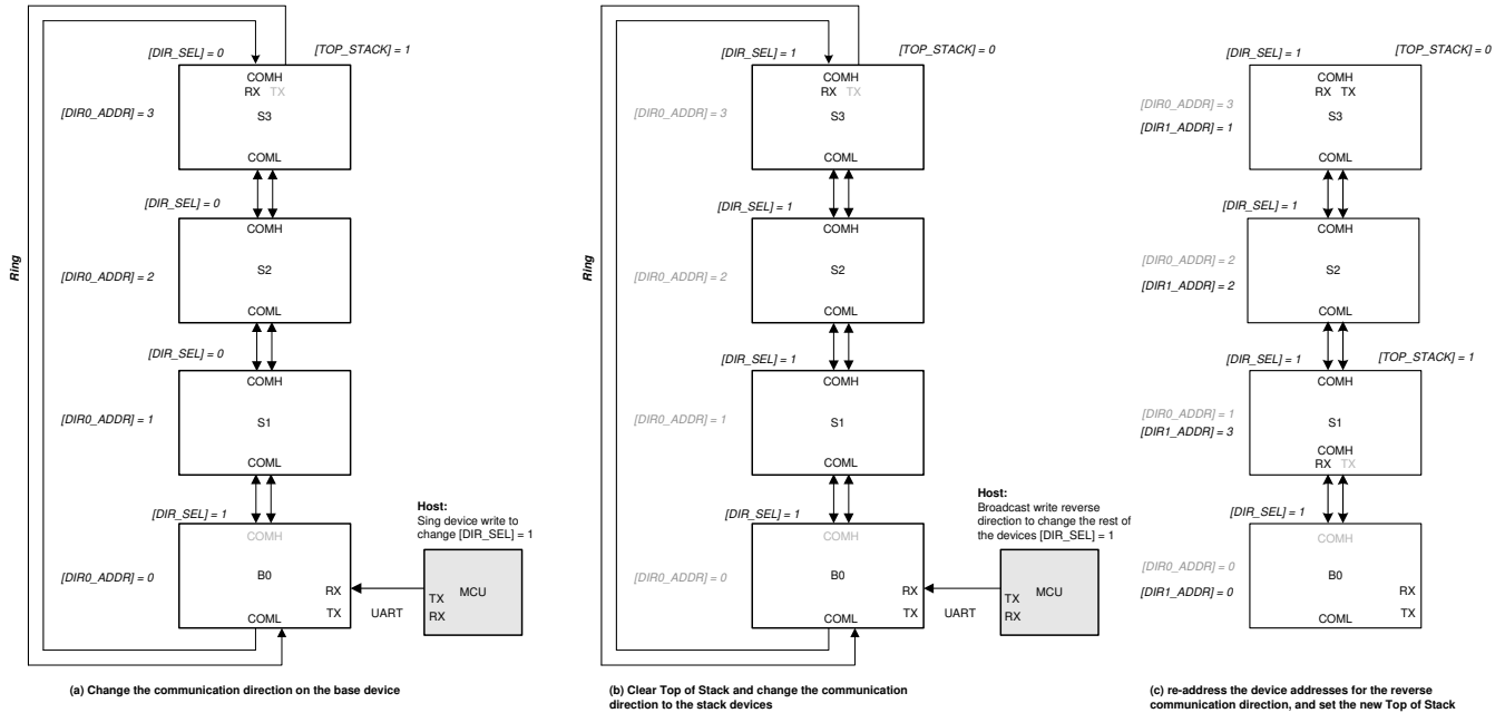
图 7-37. 更改菊花链中的通信方向的示例
