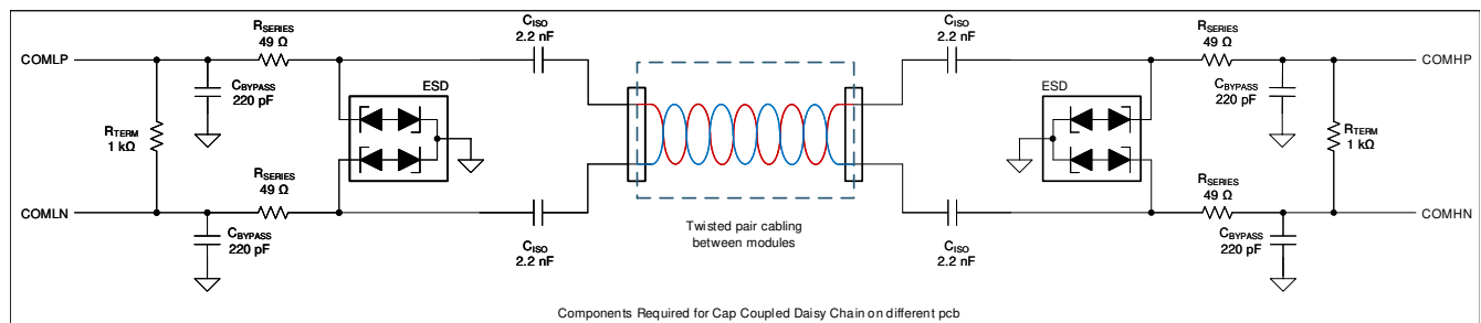
图 8-7. 不同 PCB 上的电容器隔离
