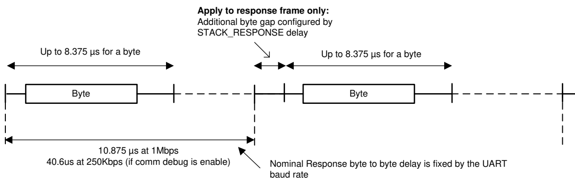
图 7-34. 菊花链字节传输
