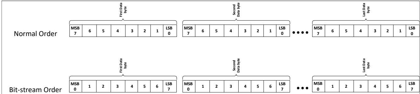
图 7-27. 位流顺序说明
