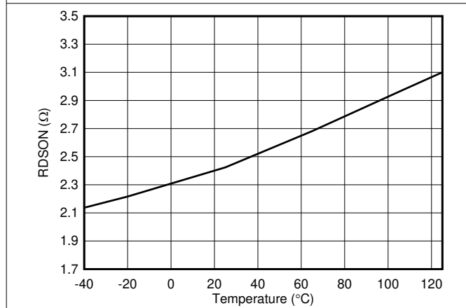
图 6-3. CBFET RDSON 与温度间的关系
