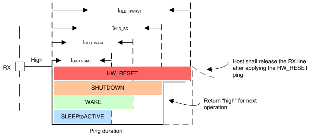
图 7-62. 通信 ping
