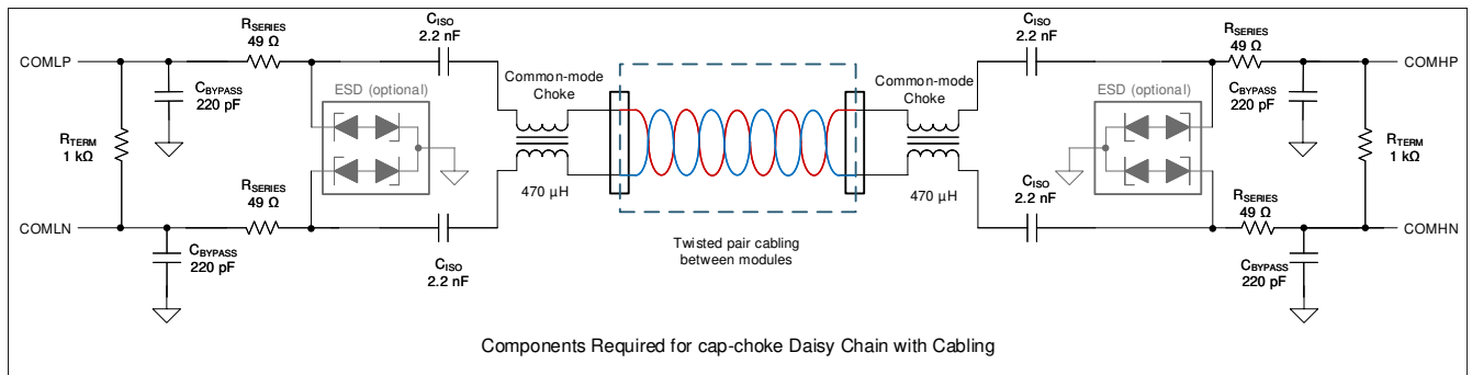
图 8-8. 电容器加扼流圈隔离
