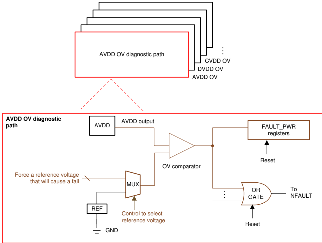
图 7-46. 电源 BIST
