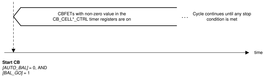
图 7-16. 手动均衡控制
