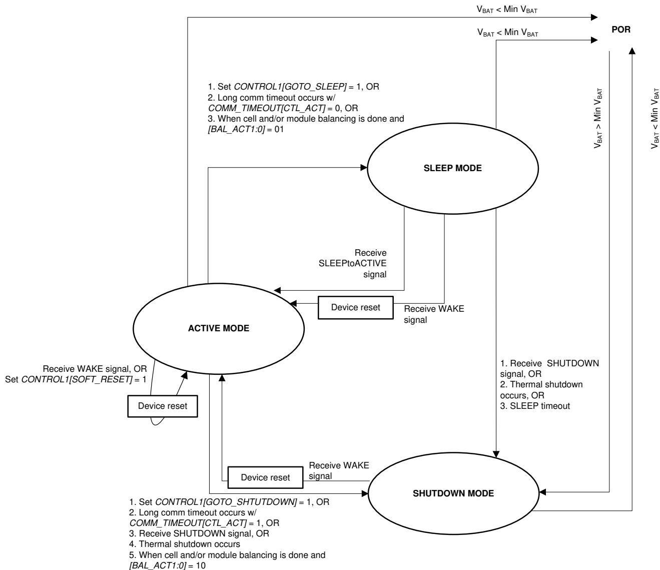
图 7-59. 功耗状态图
