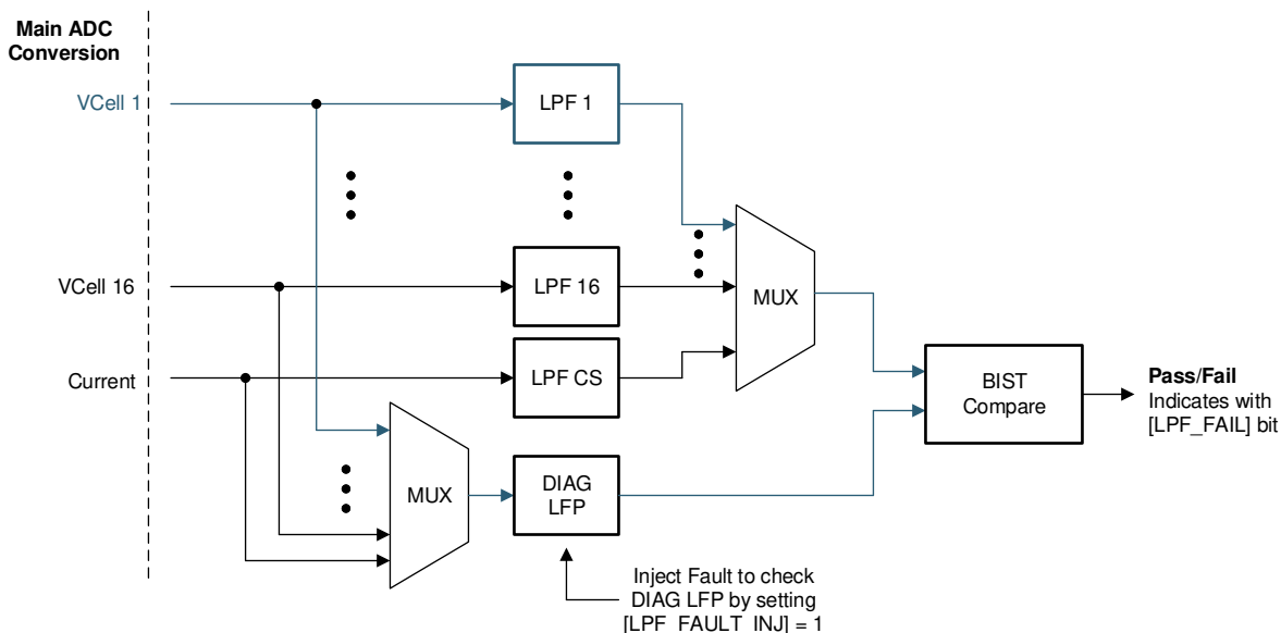
图 7-48. 后 ADC LPF 诊断 (蓝色路径是检查 LPF1 的示例)
