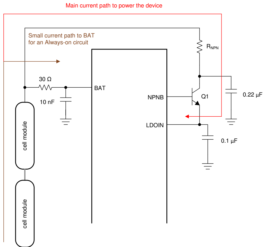
图 9-2. 器件可由堆栈中的多个电芯模块供电
