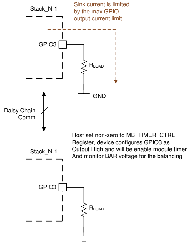
图 7-18. 模块均衡
