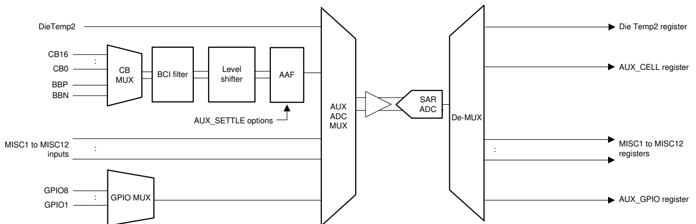
图 7-8. AUX ADC 测量路径
