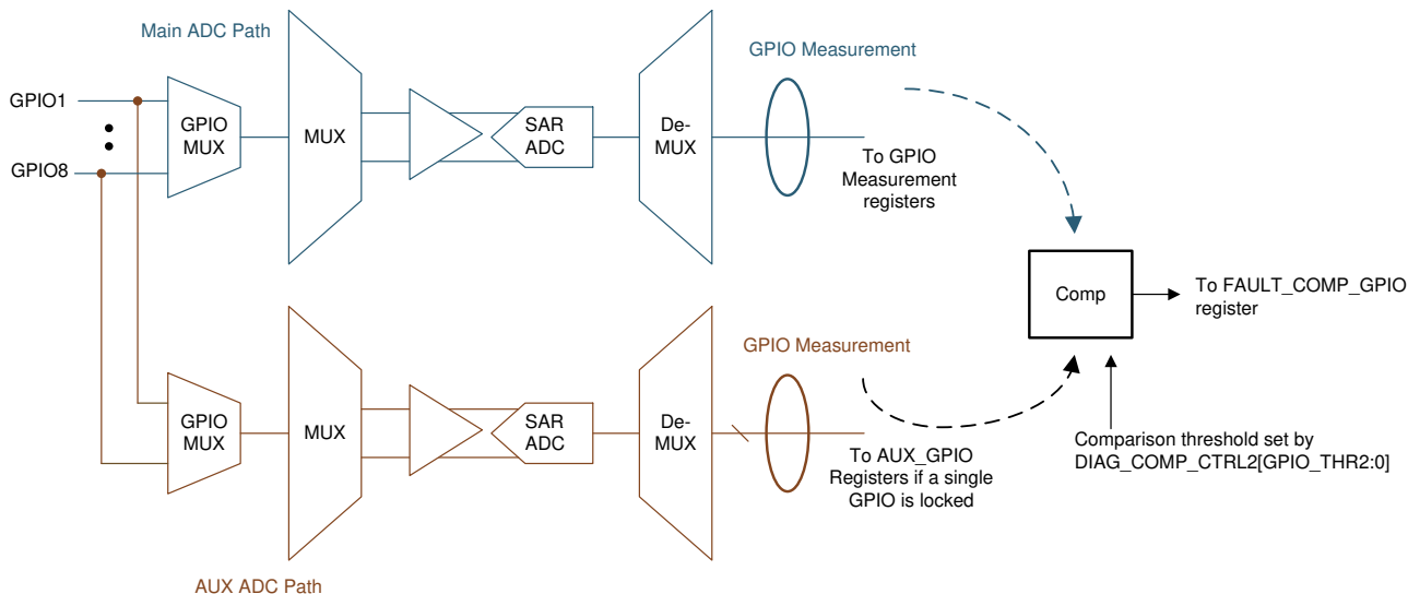
图 7-49. 热敏电阻温度 (GPIO) 测量诊断
