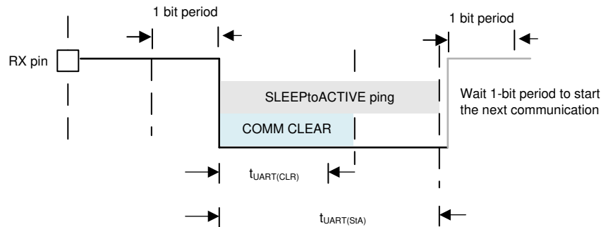
图 7-26. UART COMM CLEAR
