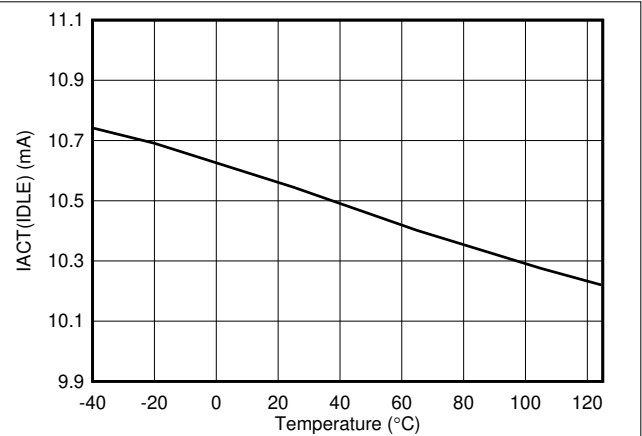
图 6-2. IACT (IDLE) 与温度之间的关系
