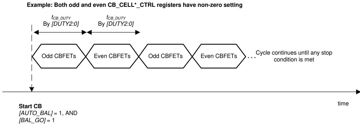
图 7-14. 自动均衡控制，示例 1
