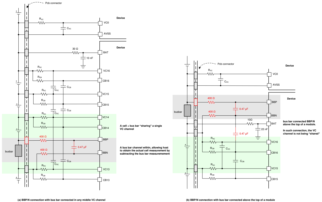
图 7-52. 连接在 BBP 和 BBN 引脚之间的汇流条
