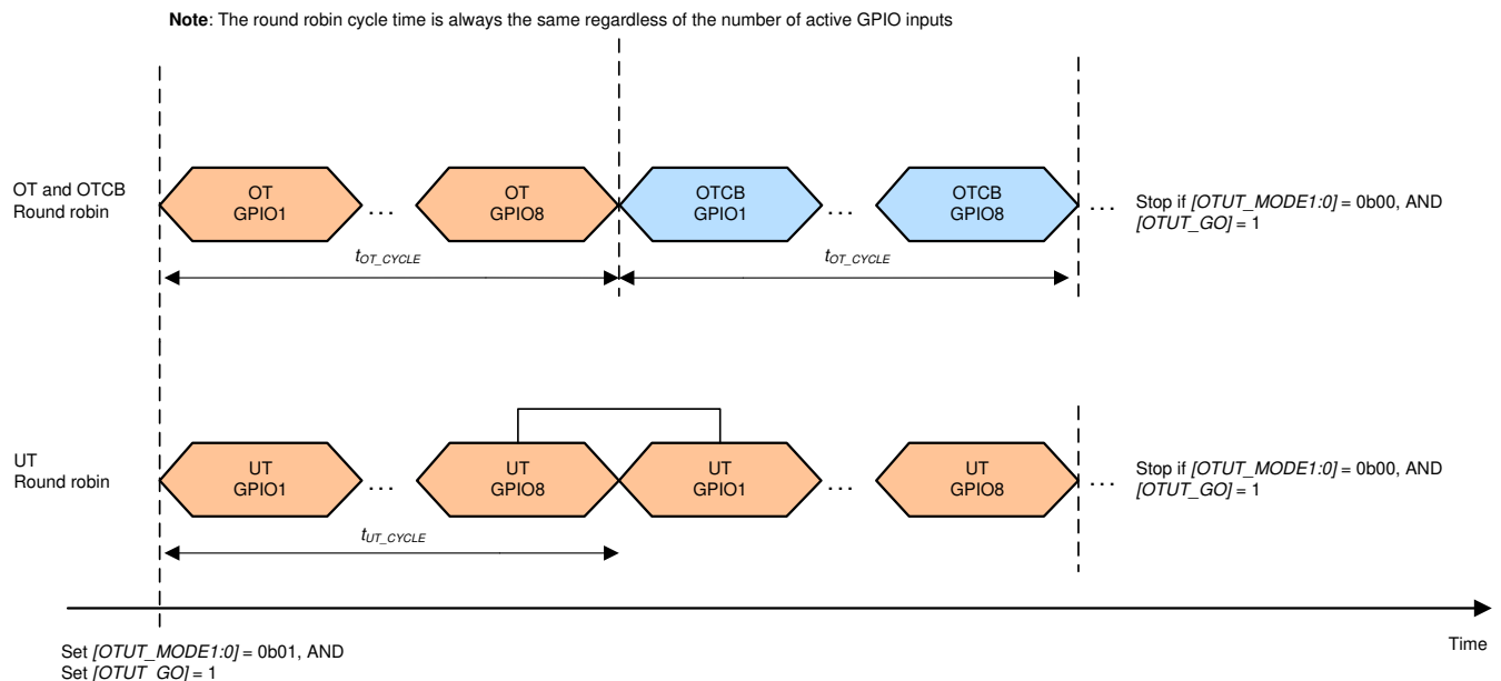
图 7-22. OT 和 UT 轮询模式
