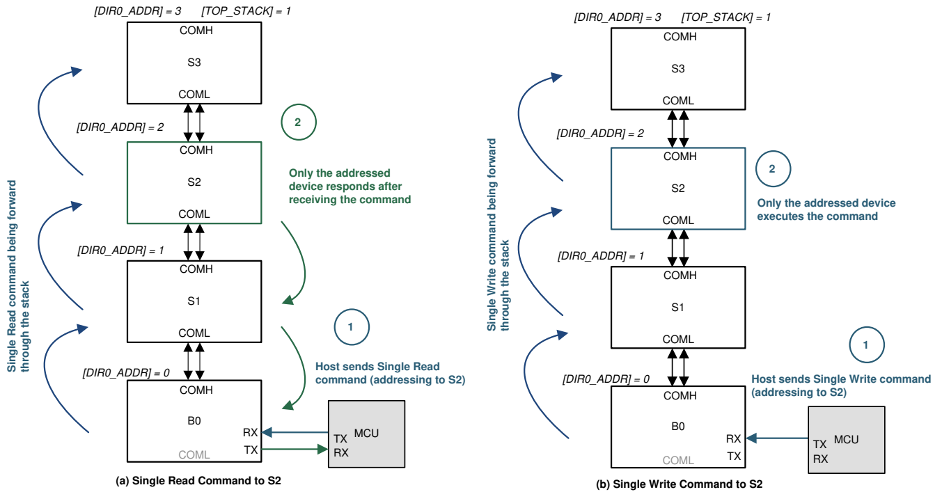
图 7-28. 单器件读取/写入
