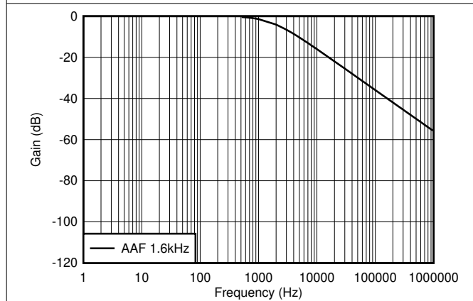
图 6-5. 主 ADC 滤波器
