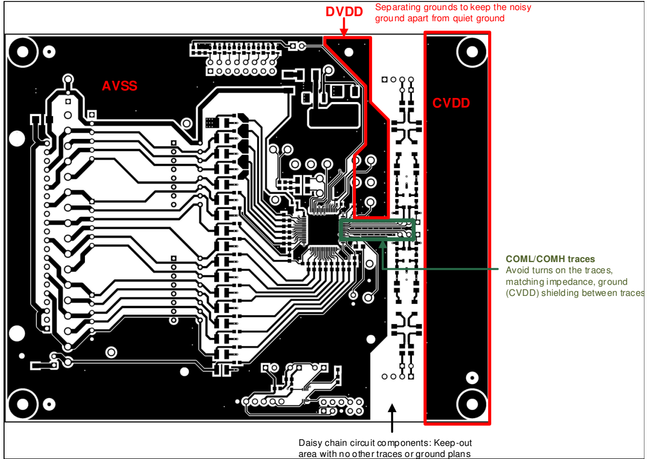
图 10-4. 顶端信号层
