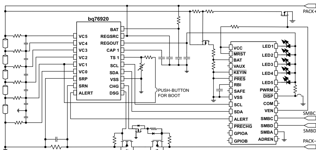
简化原理图
