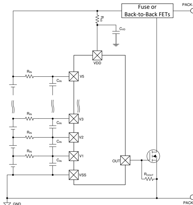
简化原理图
