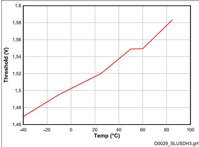
图 6-18. LD 唤醒电压与温度间的关系
