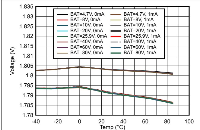
图 6-20. 不同 BAT 电平下 REG18 电压与温度间的关系
