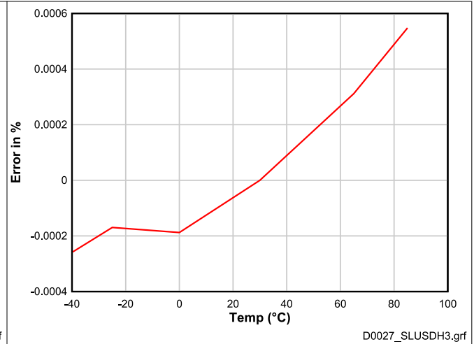
图 6-17. 库仑计增益误差与温度间的关系
