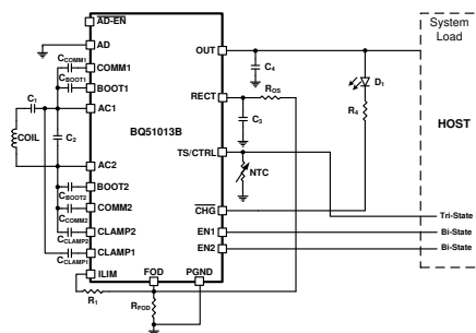
简化原理图
