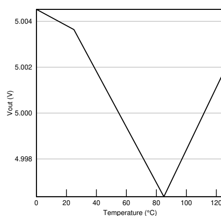
图 7-8. V_{OUT} vs Temperature
