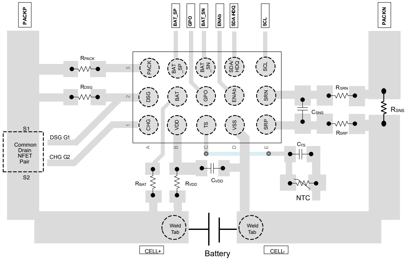
图 7-6. BQ27Z758 主要布线电路板布局布线
