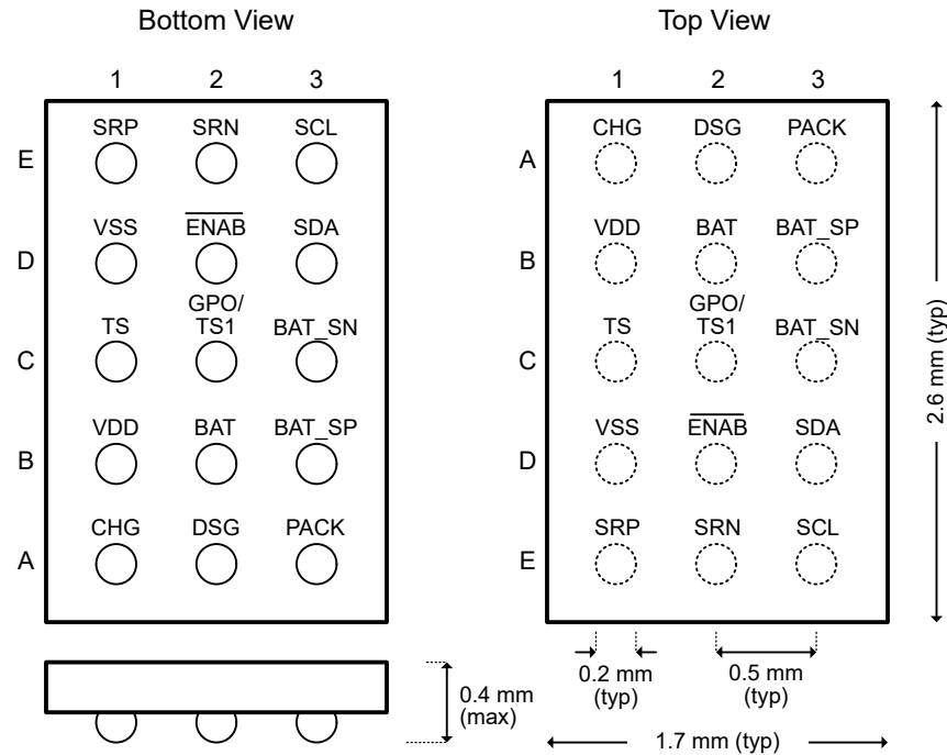
图 4-1. 引脚排列图
