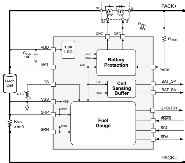
BQ27Z758 简化原理图
