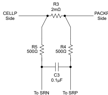
图 7-5. 用于降低 ESD 的具有推荐的 500 \Omega 电阻器的库仑计滤波器
