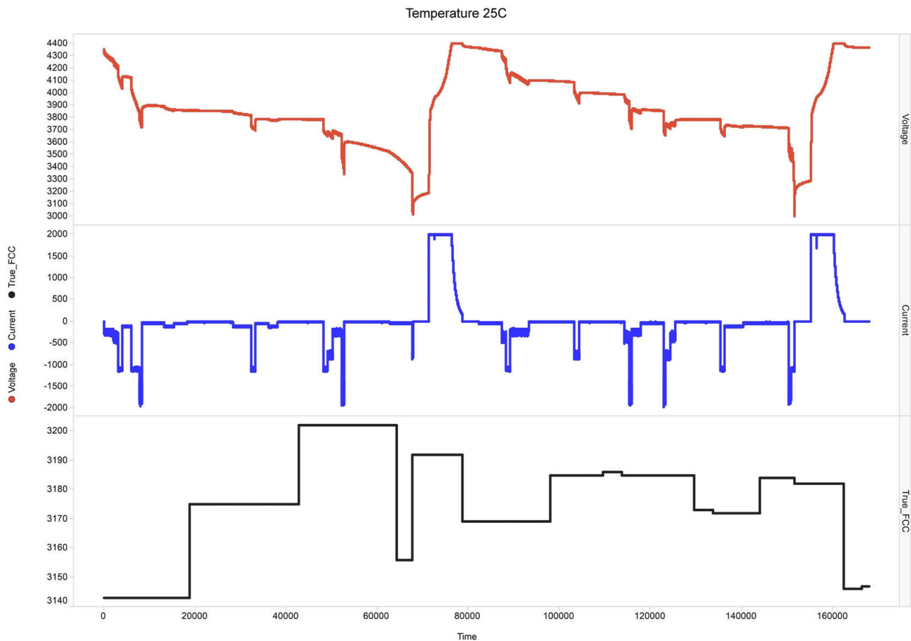
图 7-4. 充满电容量跟踪 (X 轴为秒)
