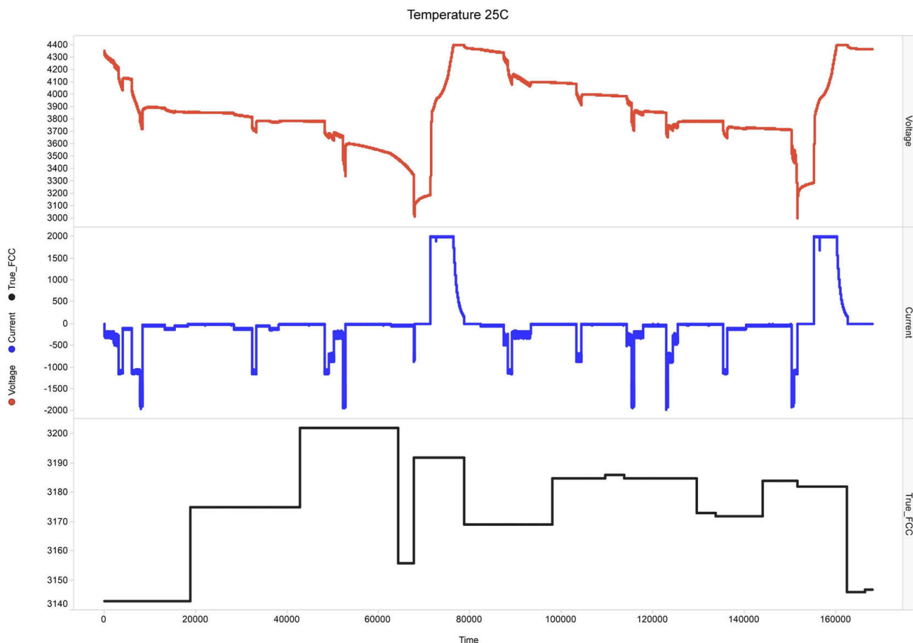
图 7-3. 充满电容量跟踪 (X 轴为秒)
