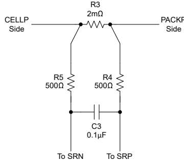
图 7-4. 用于降低 ESD 的具有推荐的 500 \Omega 电阻器的库仑计滤波器
