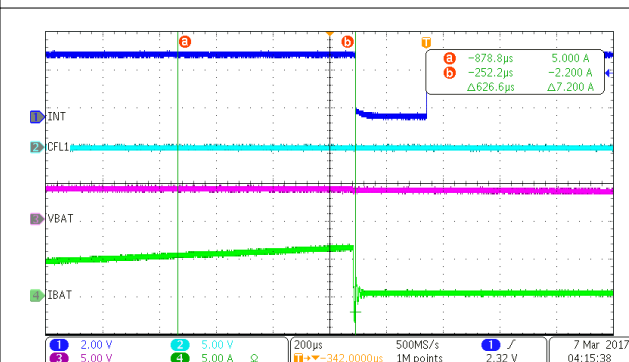
图 10-5. IBAT_OCP
