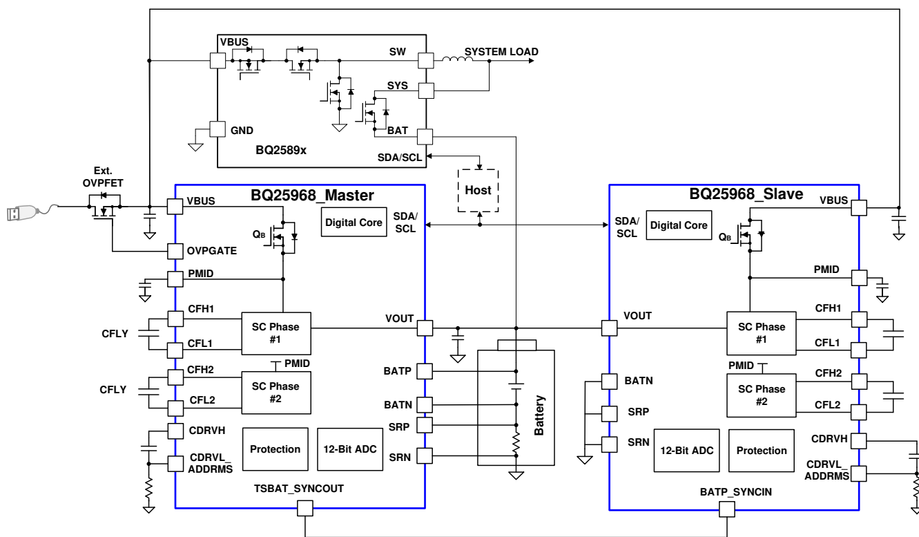
图 10-8. Parallel BQ25968 System
