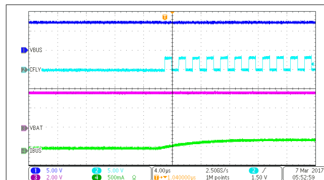
图 10-2. Power Up
