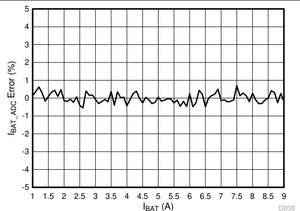
图 8-14. I_{BAT\_ADC} Error
