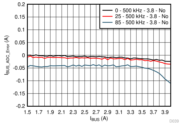
图 8-12. I_{BUS\_ADC} Error
