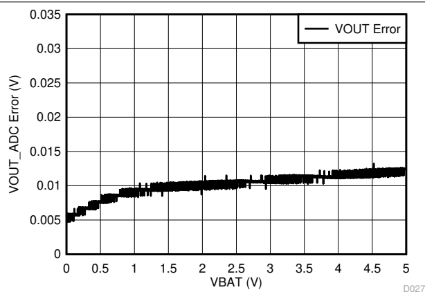
图 8-9. VOUT_ADC Error
