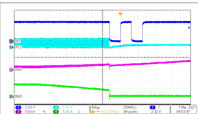
图 10-7. VBAT_OVP
