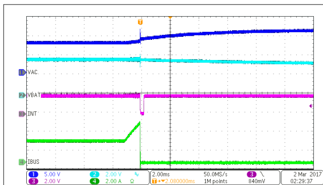
图 10-6. IBUS_OCP
