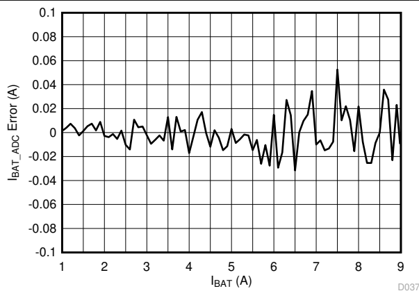
图 8-13. I_{BAT\_ADC} Error
