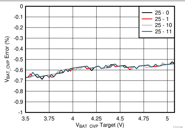
图 8-10. VBAT_OVP Error
