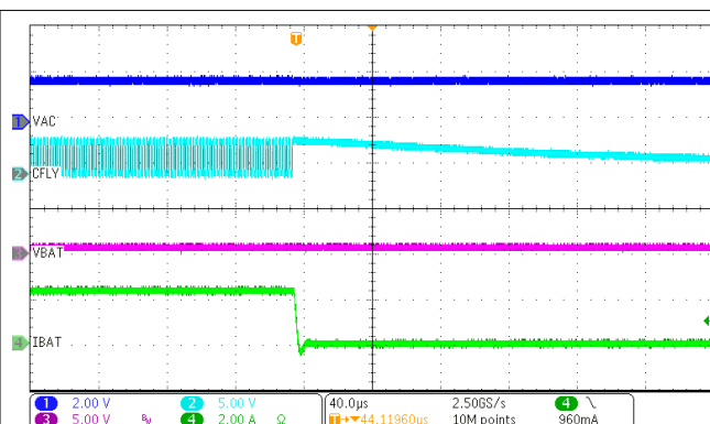
图 10-3. Disable Charge
