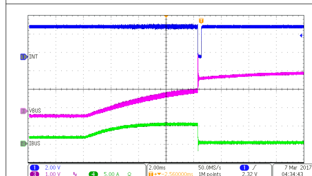
图 10-4. VBUS_OVP
