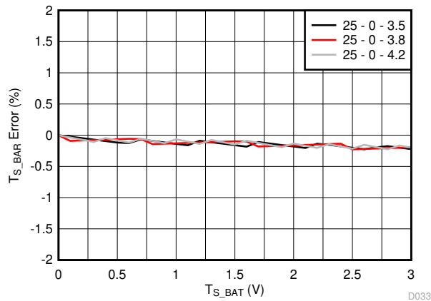
图 8-11. T_{S\_BAT} Error
