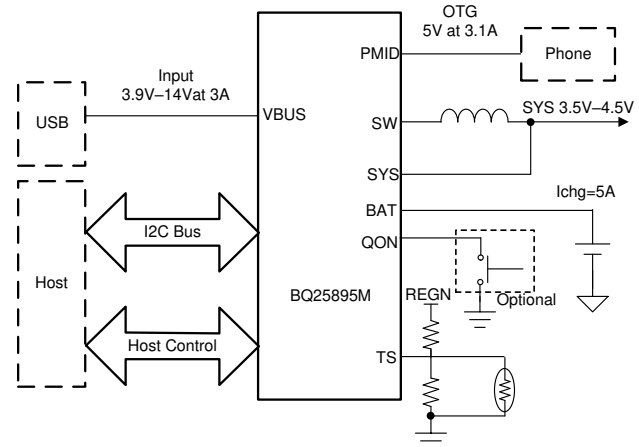
简化原理图
