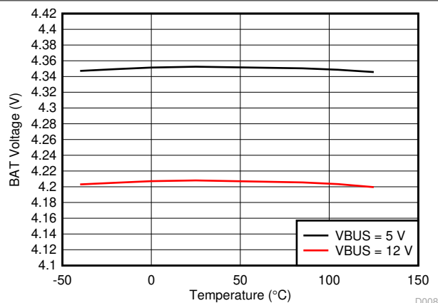
图 8-7. BAT Voltage vs Temperature
