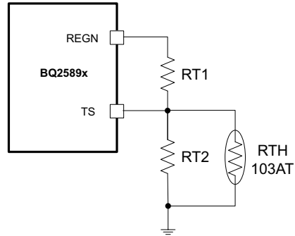
图 9-6. TS Resistor Network
