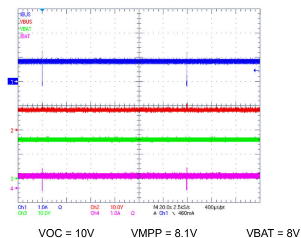
图 10-18. MPPT Operation
