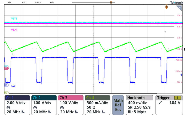
图 8-7. 经由 \overline{CE} 引脚禁用充电
