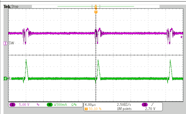
图 10-9. Charge Enable
