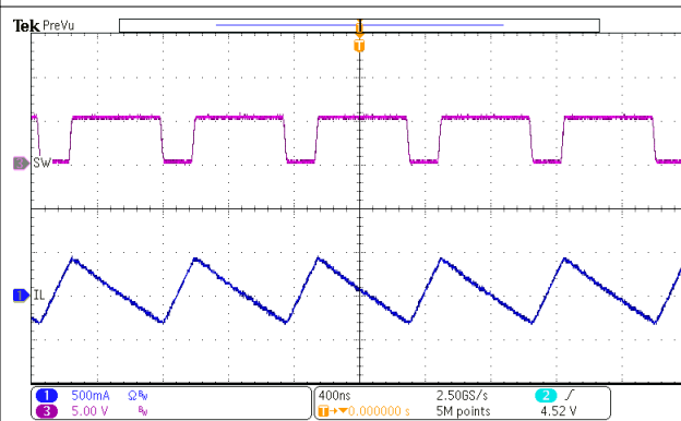
图 10-11. OTG Switching
