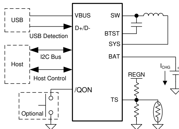
简化版应用
