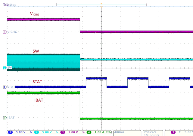
图 9-6. ICHG 引脚短路保护
