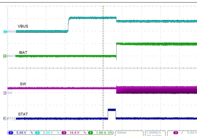
图 9-3. 充电周期
