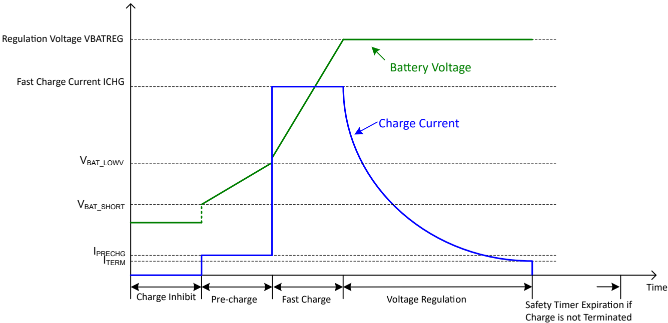
图 8-1. 电池充电曲线
