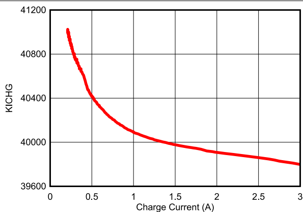
图 7-3. KICHG 与充电电流间的关系
