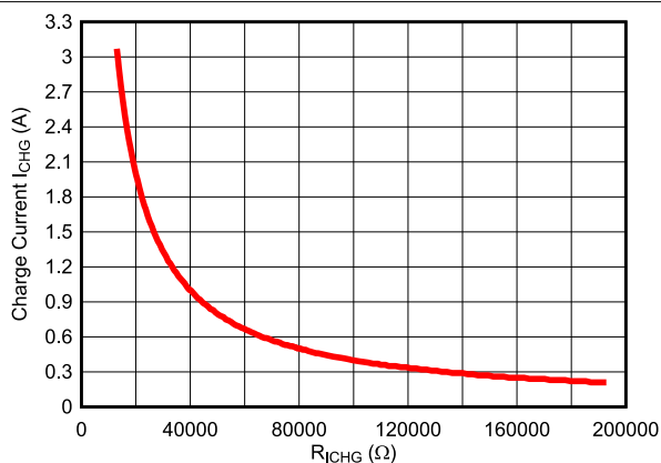
图 7-4. 充电电流与充电电流设置电阻 R_{ICHG} 间的关系
