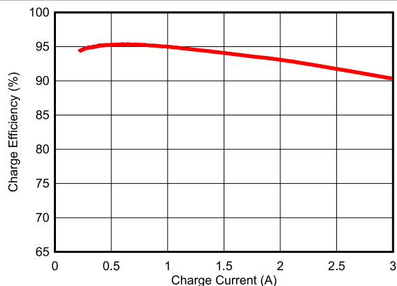
图 7-1. 1 节电池充电效率与充电电流间的关系
