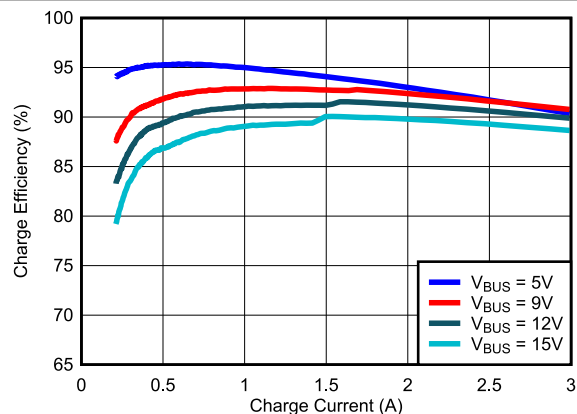
图 7-2. 1 节电池充电效率与充电电流间的关系
