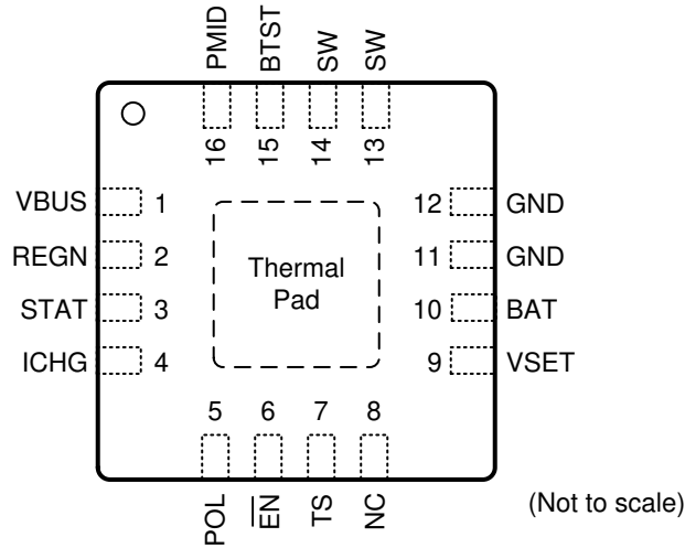
图 6-1. RTE 封装 16 引脚 WQFN 顶视图
