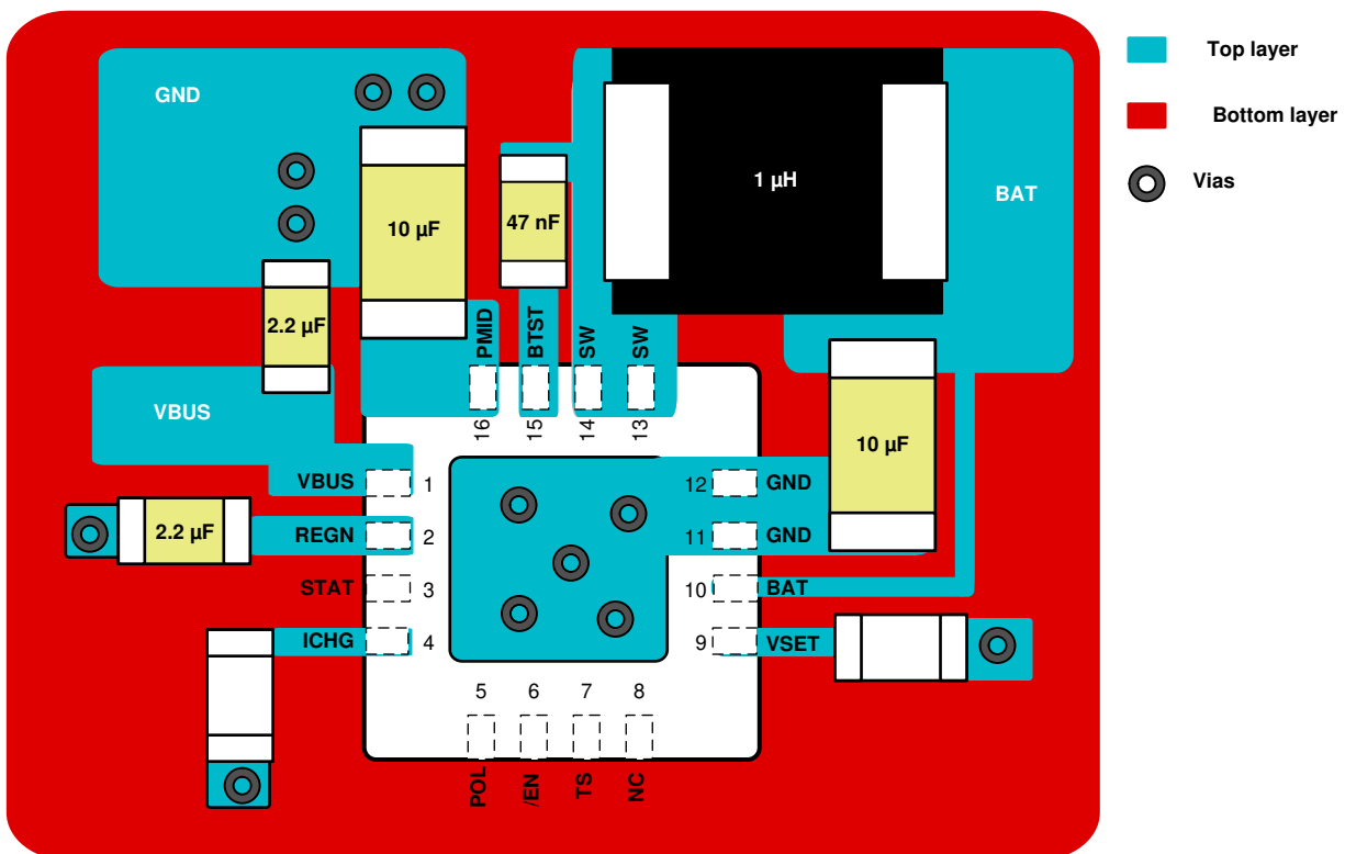
图 11-2. 布局示例
