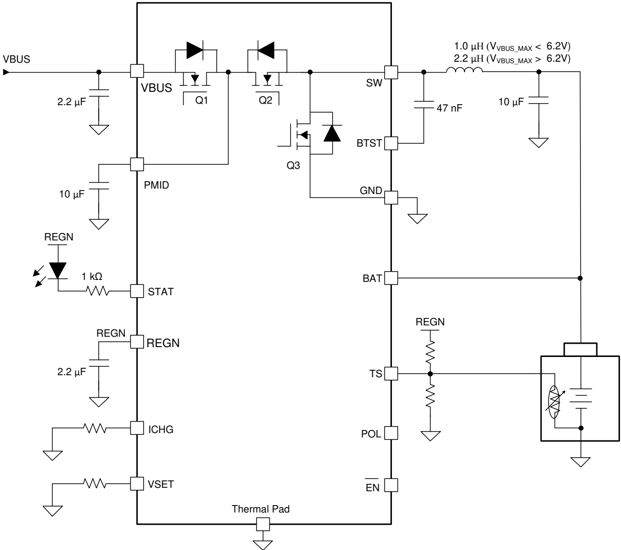
图 9-1. 典型应用图
