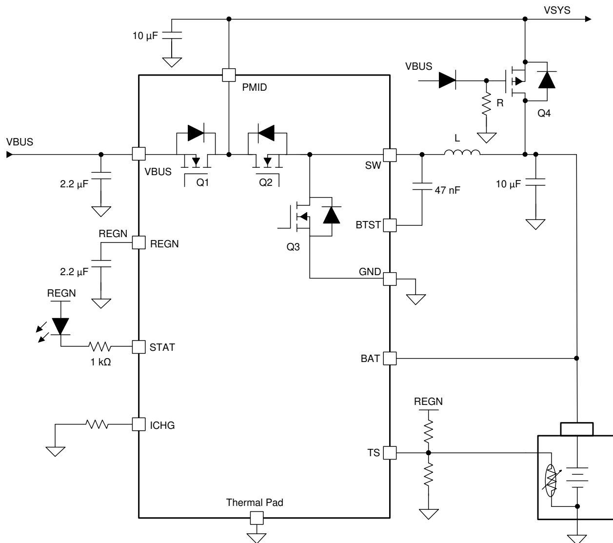
图 9-7. 电源路径典型应用图
