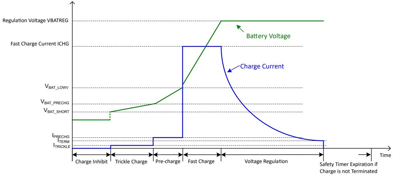
图 8-2. V_{BATREG} = 3.6V 时的电池充电曲线
