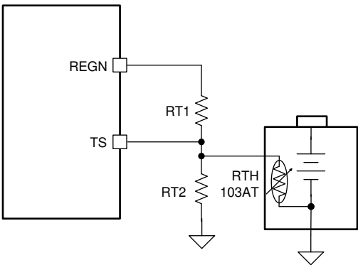
图 8-3. 电池温度检测电路
