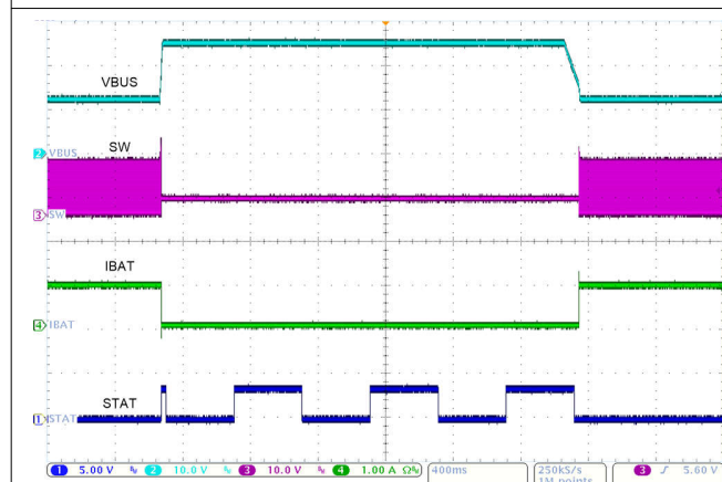
图 9-2. 从 VBUS 上电
