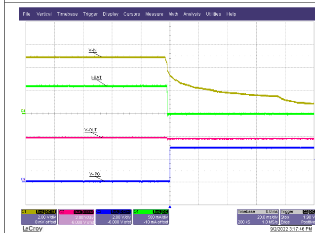
图 8-2. 在有电池的情况下上电
