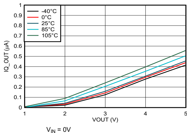
图 6-9. 输出静态电流与输出电压间的关系
