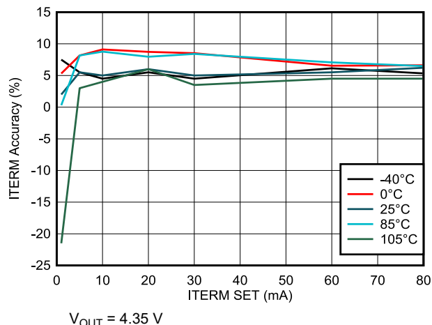
图 6-10. 终止电流精度与终止电流设置间的关系
