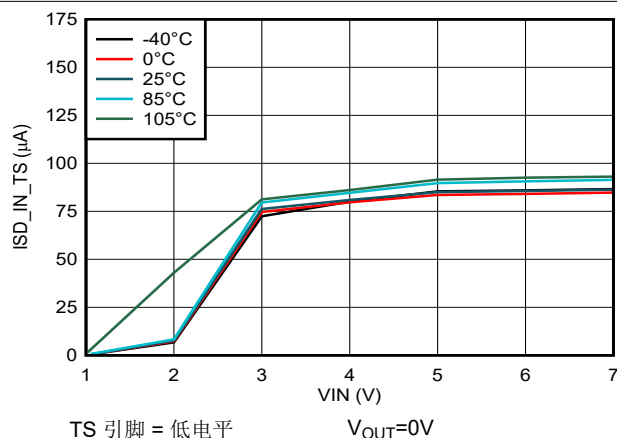
图 6-7. 输入关断电流与输入电压间的关系
