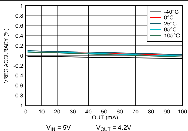
图 6-2. 负载调整率
