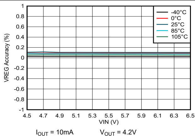
图 6-1. 线性调整率
