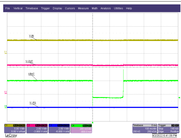
图 8-3. 在没有电池的情况下上电
