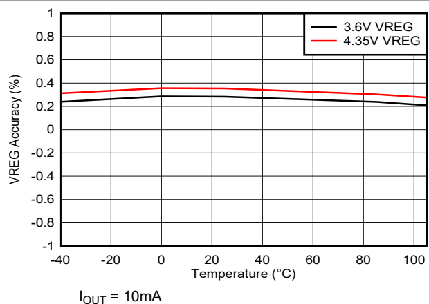
图 6-5. VSET 精度与温度间的关系
