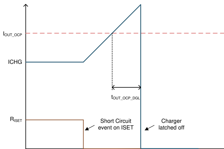
图 7-4. 过流保护
