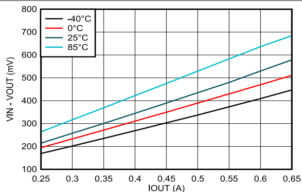
图 6-6. 压降电压与输出电流间的关系
