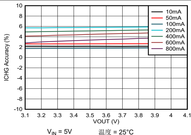
图 6-3. ICHG 精度与 V_{OUT} 间的关系
