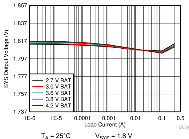
图 10-15. 1.8 V_{\text{SYS}} Load Regulation
