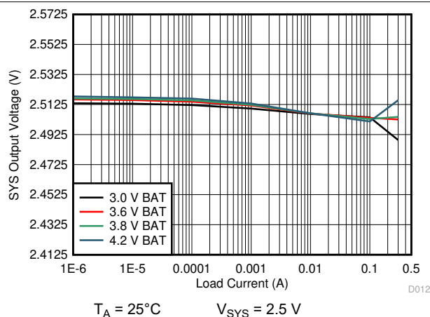
图 10-16. 2.5 V_{\text{SYS}} Load Regulation
