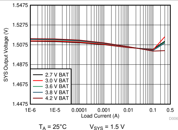
图 10-14. 1.5 V_{\text{SYS}} Load Regulation
