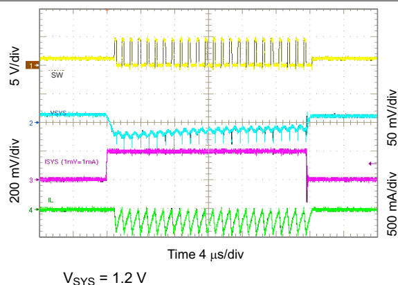
图 10-36. 1.2 V_{SYS} Load Transient, 0 to 200 mA
