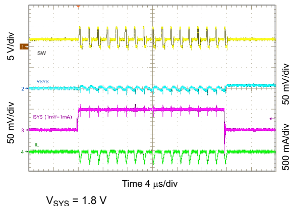
图 10-32. 1.8 V_{SYS} Load Transient, 0 to 50 mA
