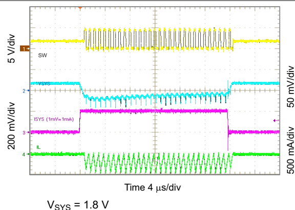
图 10-37. 1.8 V_{SYS} Load Transient, 0 to 200 mA
