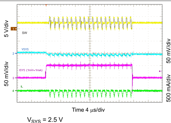
图 10-34. 2.5 V_{SYS} Load Transient, 0 to 50 mA
