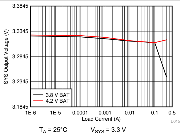
图 10-17. 3.3 V_{\text{SYS}} Load Regulation
