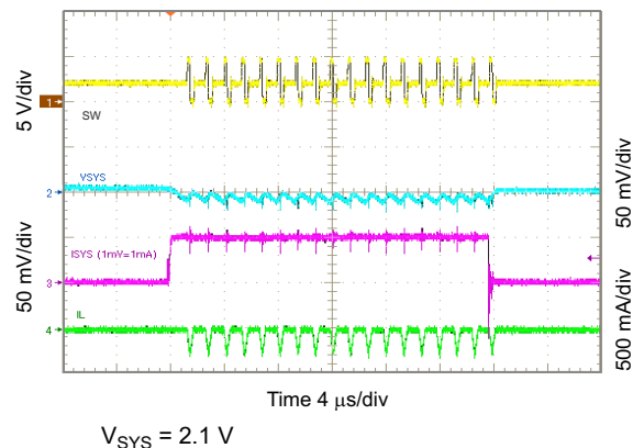
图 10-33. 2.1 V_{SYS} Load Transient, 0 to 50 mA
