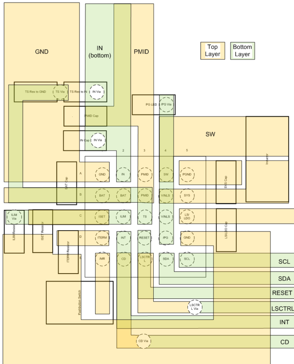
图 12-1. BQ25125 Layout
