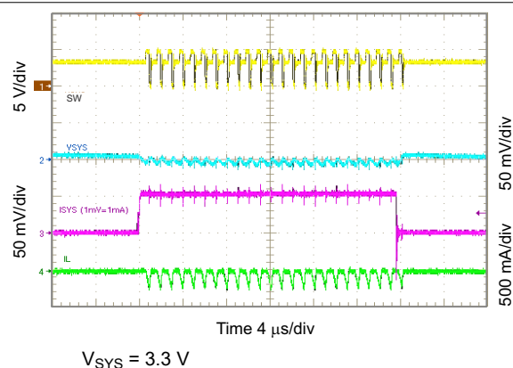
图 10-35. 3.3 V_{SYS} Load Transient, 0 to 50 mA
