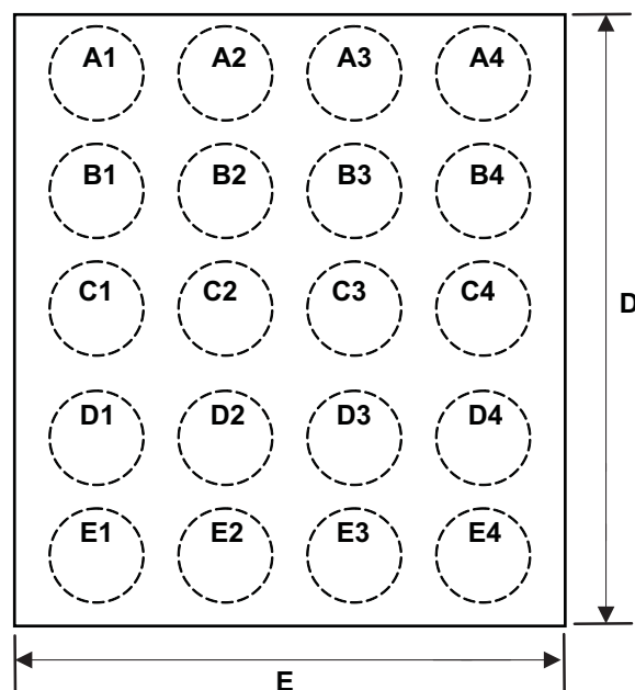
WCSP PACKAGE (Top View)
