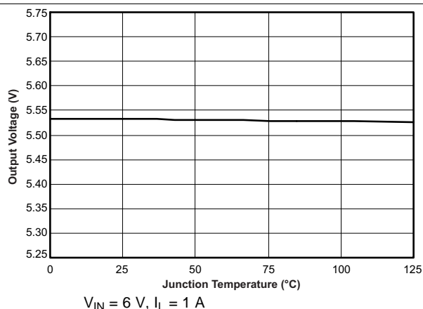
图 9. Output Regulation Voltage vs Temperature - bq24079QW-Q1
