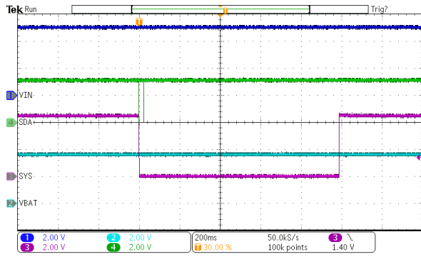
图 8-8. 通过 I 2 C 进行硬件复位
