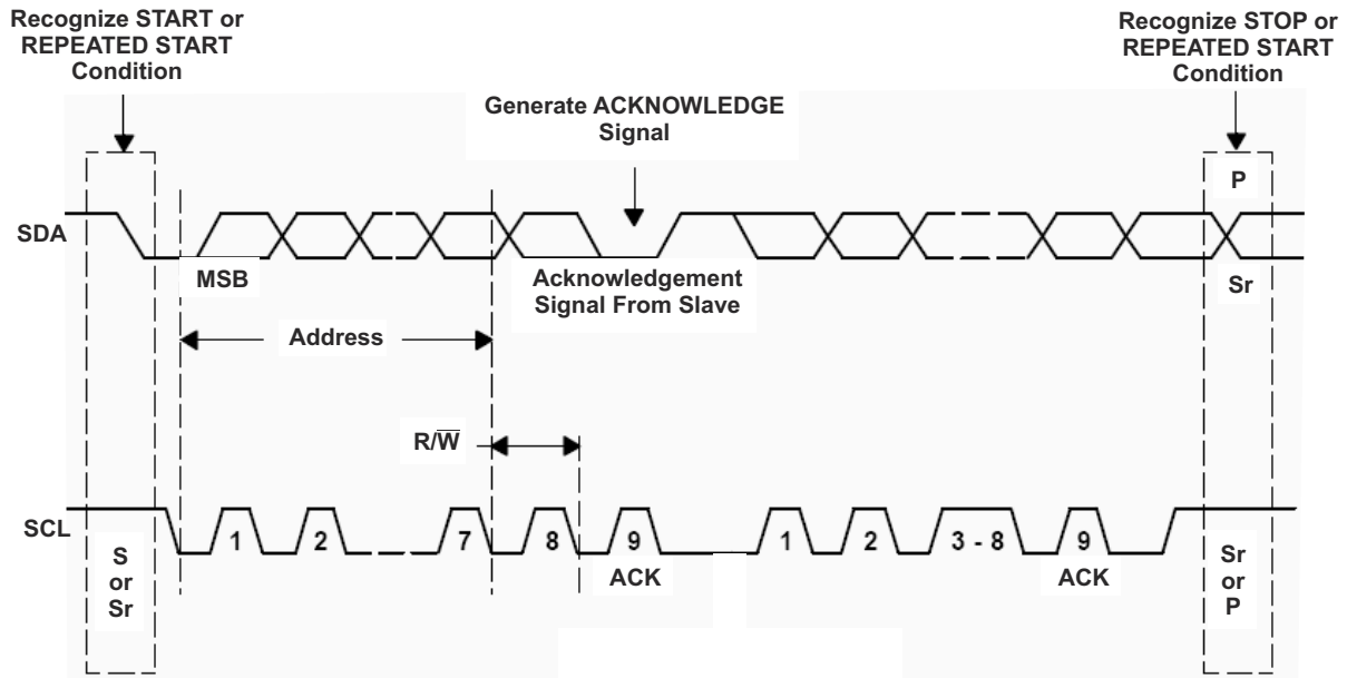
图 7-7. 总线协议
